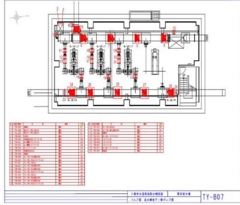
水道施設台帳設備平面図（抜粋）
