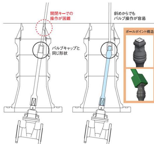
ボールポイント構造の説明
