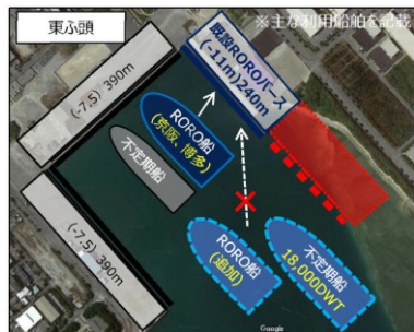
▲中城湾港整備イメージ
