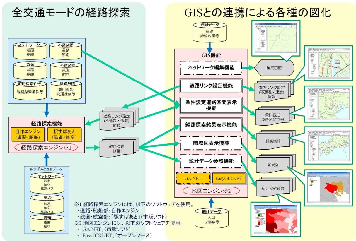
図ー1 システム構成(NITAS Ver.2.8)
