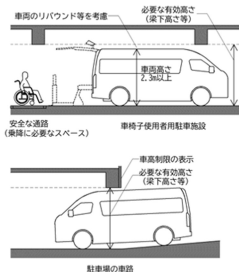
図3.4.15 車椅子使用者用駐車施設等(屋内)における有効高さのイメージ
