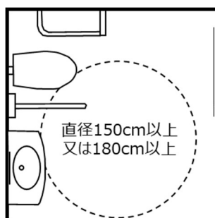
図 3.4.2 バリアフリートイレにおける車椅子の転回スペース
