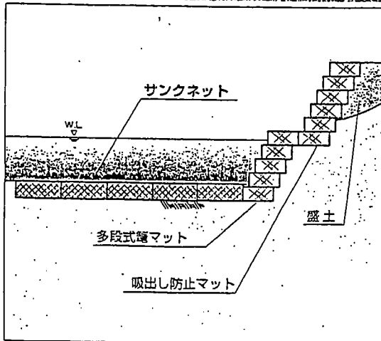
北海道開発局 小樽開発建設部(尻別川) 根固め工 SN-2
