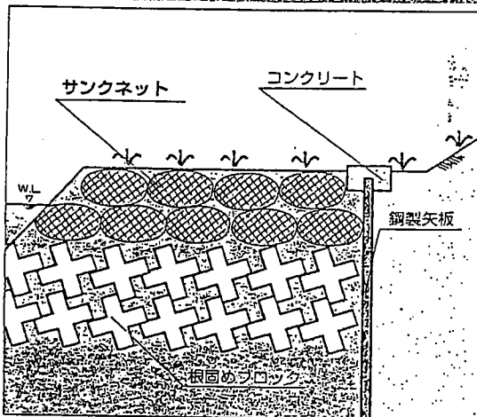
北海道開発局 小樽開発建設部(尻別川) 根固め工 SN-2
