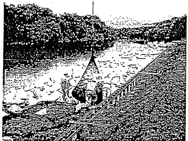
北海道開発局 小樽開発建設部(尻別川) 根固め工 SN-2
