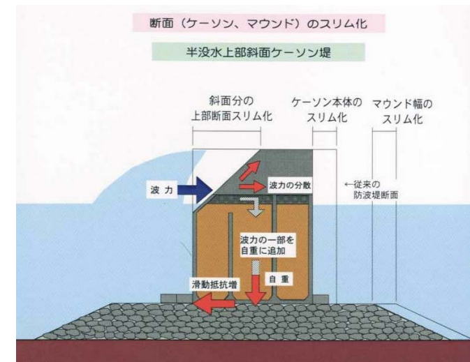
〔半没水上部斜面ケーソン堤〕
