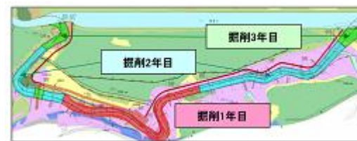
(新) 鋼矢板締切方式
