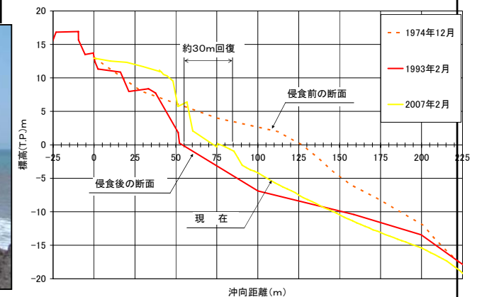
【断面変化図 富士海岸 No48_000】
