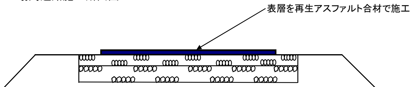
場周道路施工断面図
