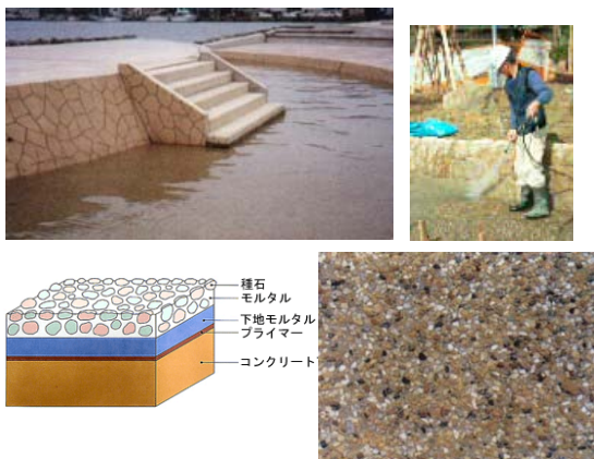
従来工法：化粧骨材洗い出し舗装
