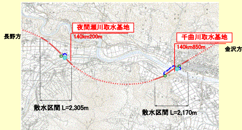
（従来）夜間瀬川・千曲川取水基地
