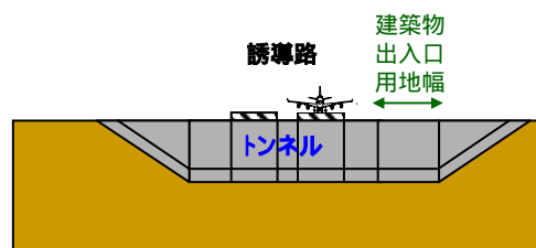
建築物移転前トンネル延長 概念図
