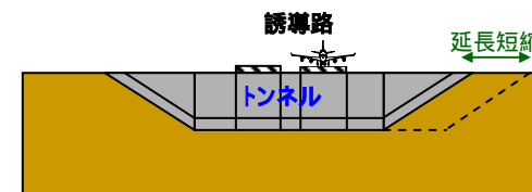
建築物移転後トンネル延長 概念図
