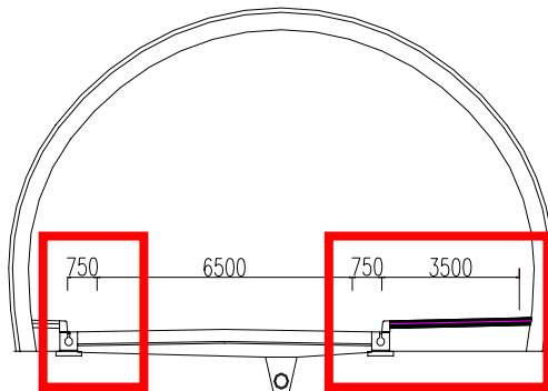
当初の断面
