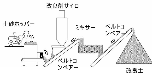
固定式ミキサ混練工法
