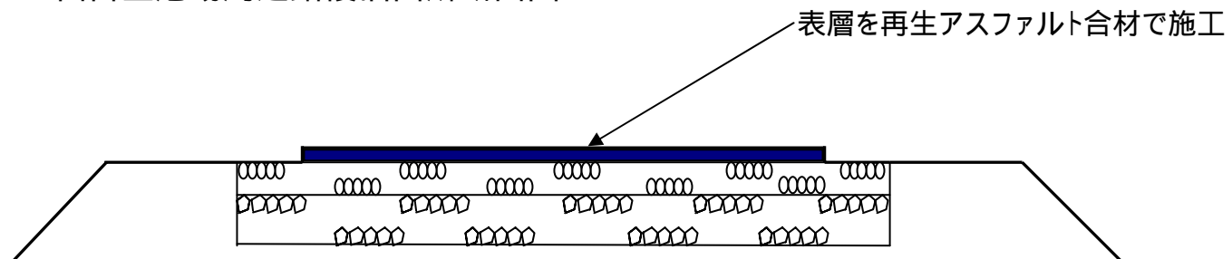
仙台空港場周道路復旧箇所断面図
