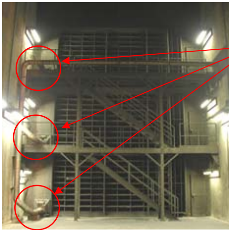
空気圧による 除塵フィルター 洗淨装置
