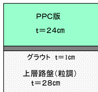
現PPC舗装
