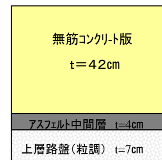
計画コンクリート舗装
