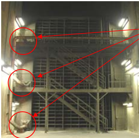
空気圧による 除塵フィルター 洗浄装置
