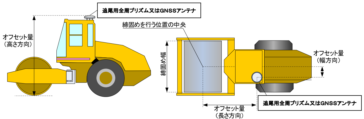
参考図4 オフセット量・締めめ幅の計測位置（土工用振動ローラを使用する場合の例）
