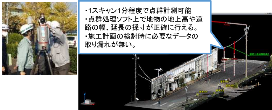
通常計測による50m先の1㎡データ
