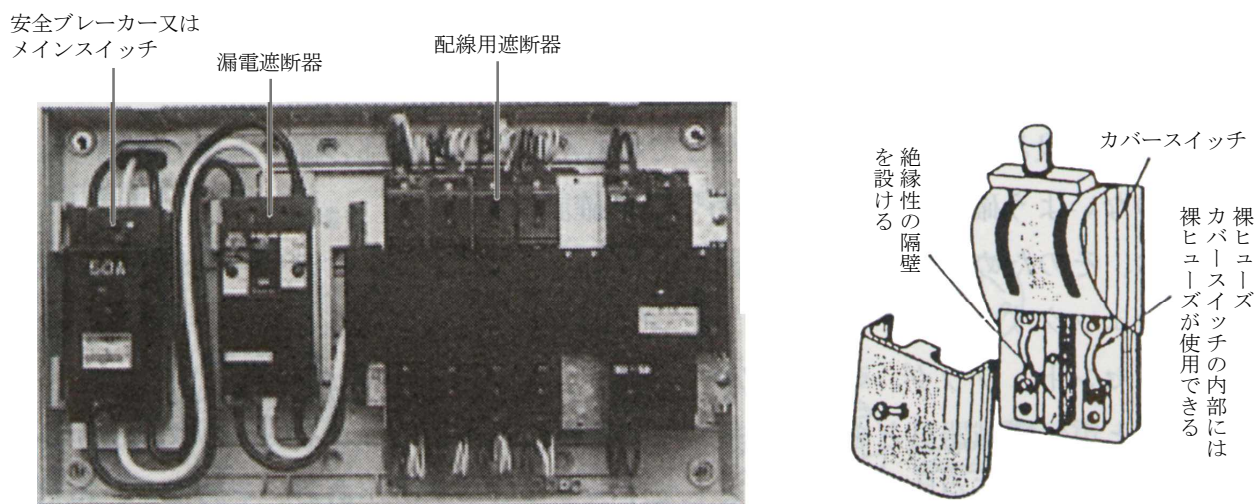
図 1 4 開閉器 (例)
