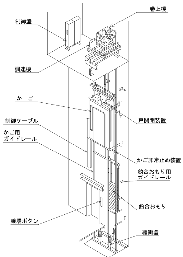
ロープ式エレベータ（機械室あり）
