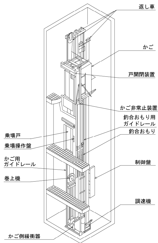
ロープ式エレベータ（機械室なし）
