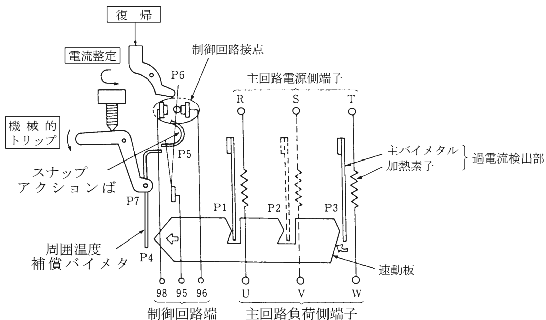
図 1 3 サーマルリレーの原理構造
