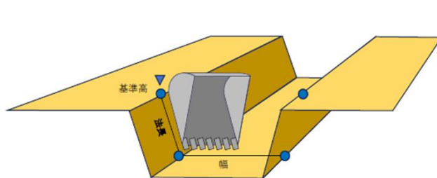
刃先位置の単点計測 (新たな計測手法)
