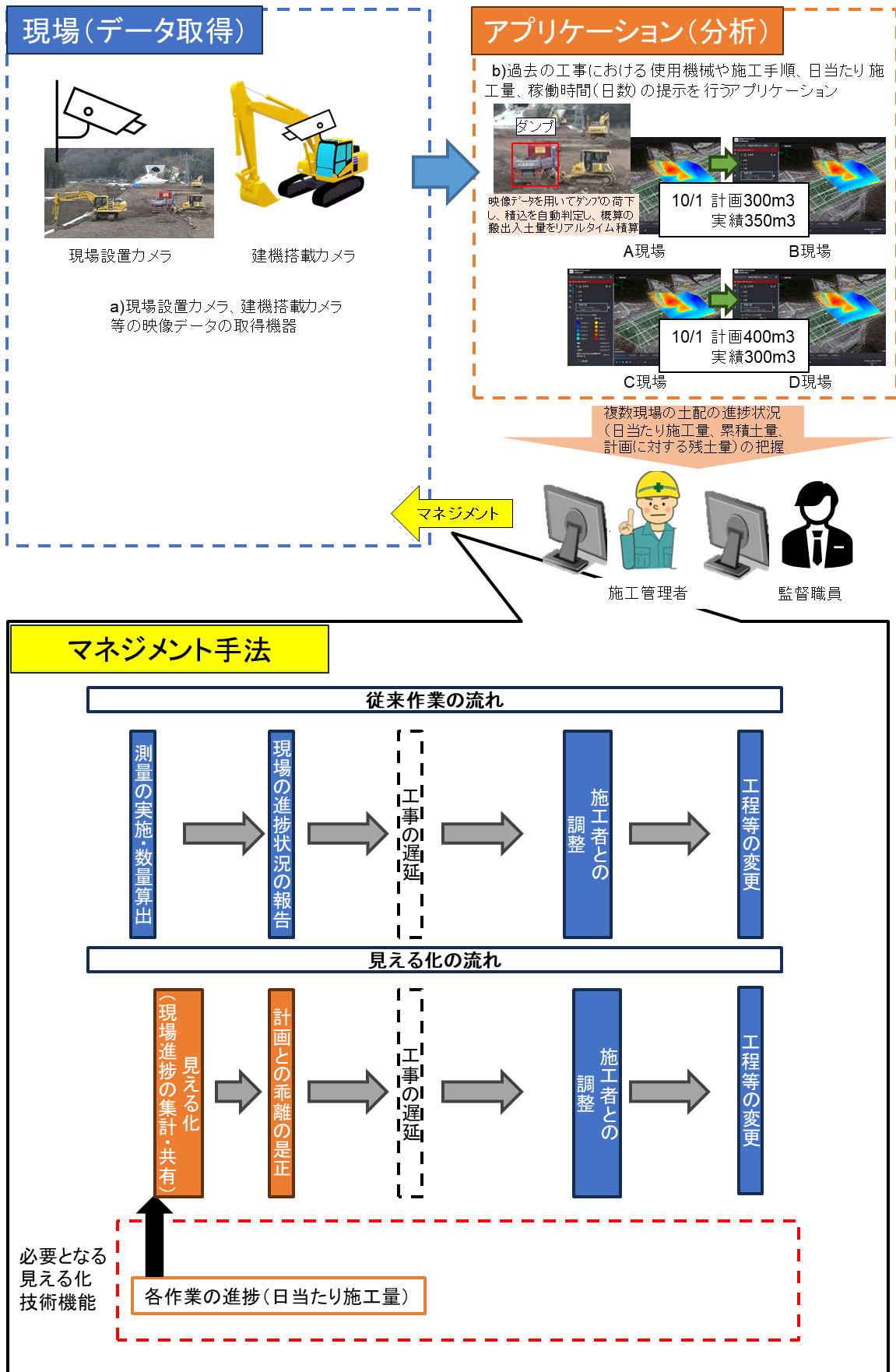
図14 工程進捗管理による実工程に適した資機材等調整(映像データ) 実施イメージ
