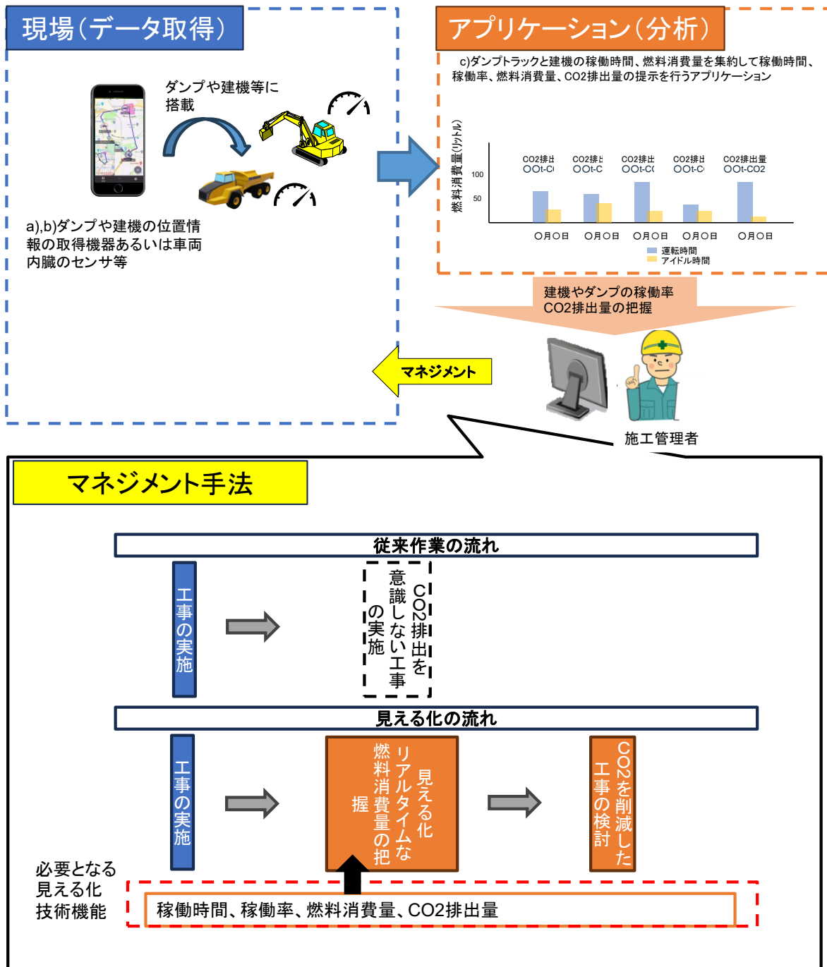
図17 CO 2 排出量の見える化による排出量削減 実施イメージ
