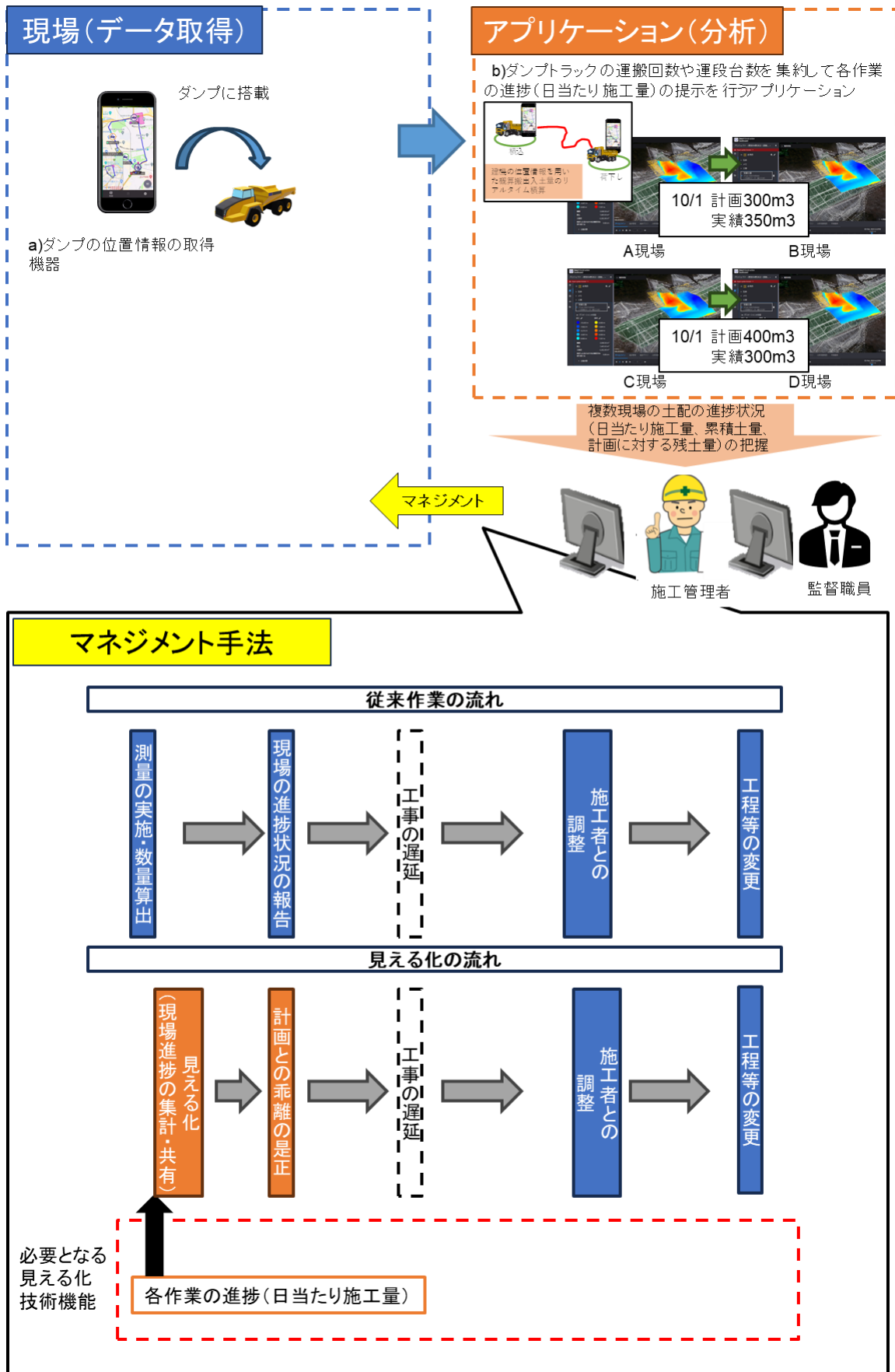
図 1 0 工程進捗管理による実工程に適した資機材等調整 (機械稼働データ) 実施イメージ
