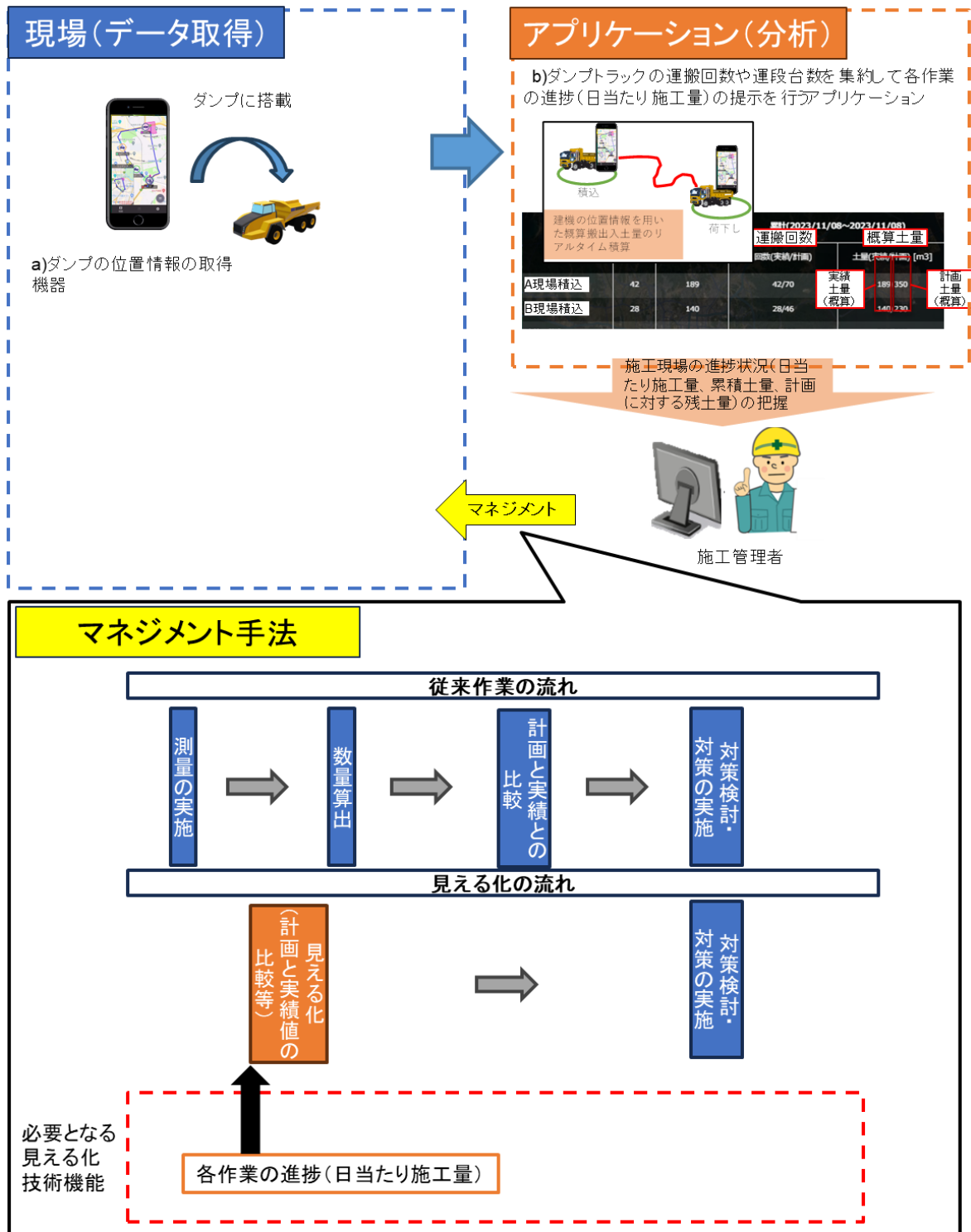
図9 工程進捗管理による実工程に適した資機材等調整（機械稼働データ） 実施イメージ
