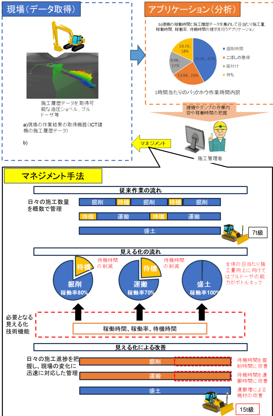
図6 稼働状況等の把握による工程の最適化(施工履歴データ) 実施イメージ
