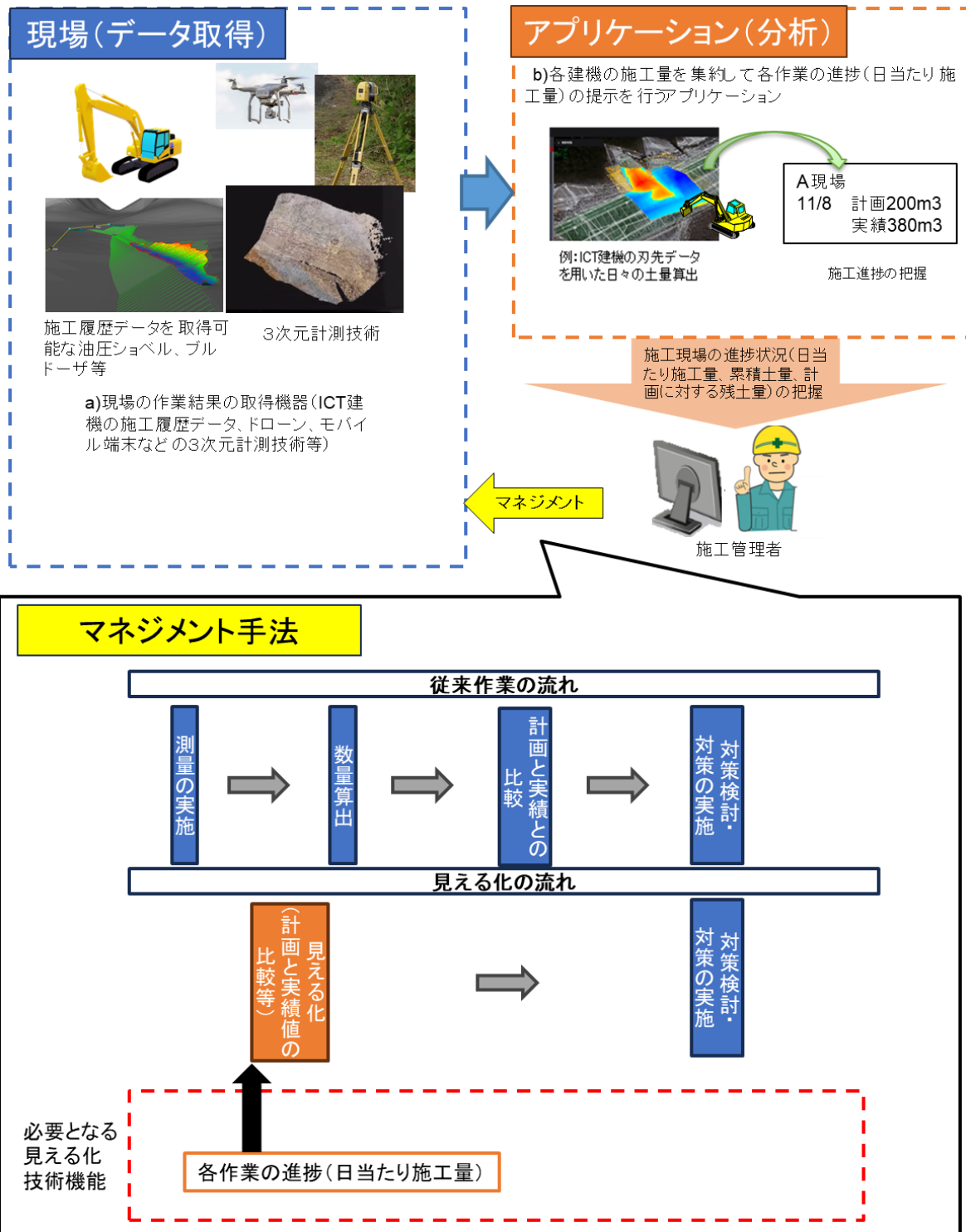
図 1 1 工程進捗管理による実工程に適した資機材等調整(施工履歴データ) 実施イメージ
