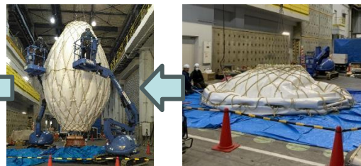
地上実証モデルの展開過程
