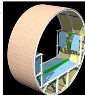
改良型与圧モジュール断面図
