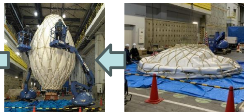
地上実証モデルの展開過程
