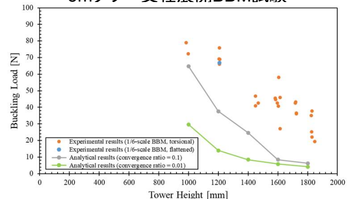
タワーの座屈試験と解析の関係
