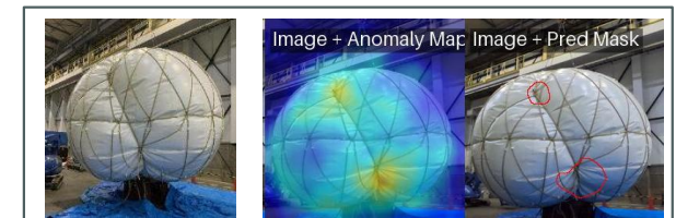
フルスケールモデルによる検知
