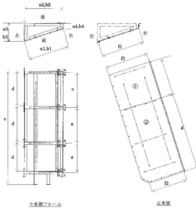
2. 止水板
