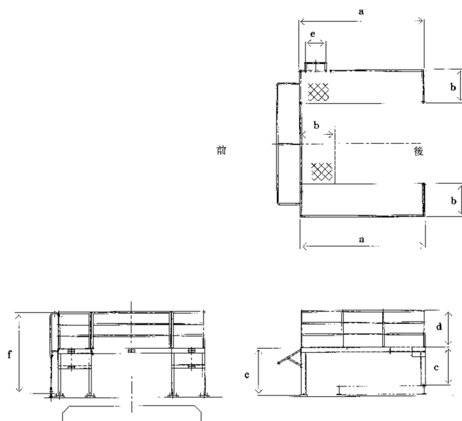
3. 架台
