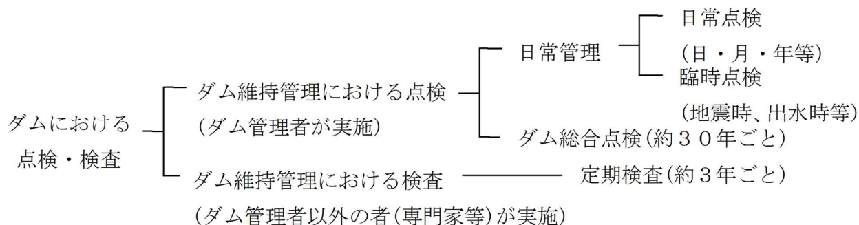
図 18 ダム維持管理における点検・検査の種類
