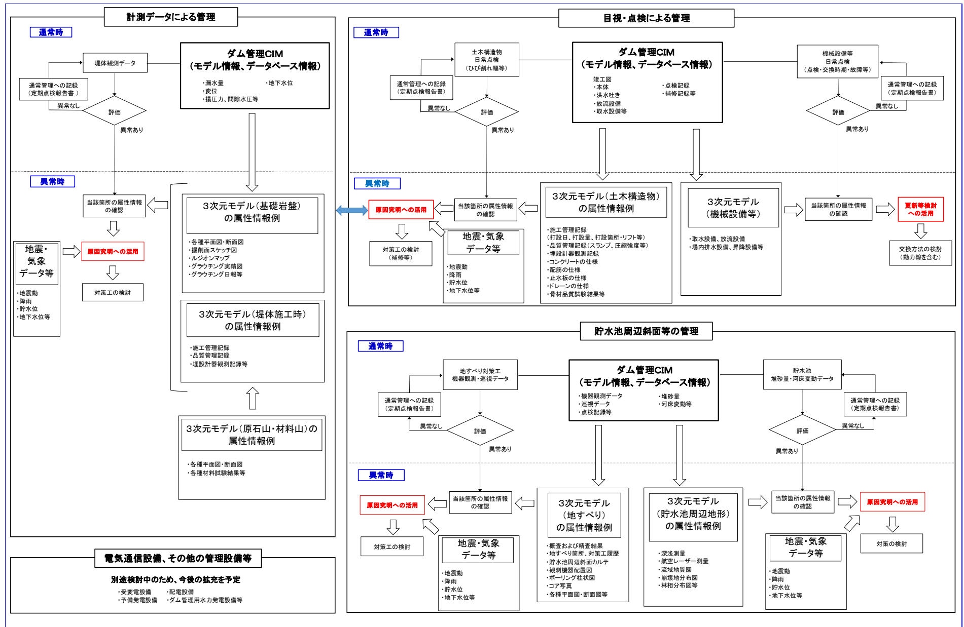
図 23 ダム管理 CIM の活用フロー（案）
