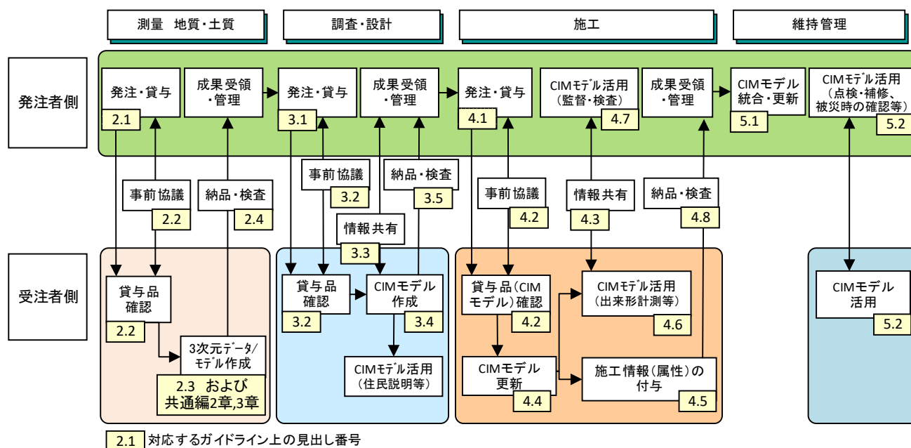
図 1 CIM モデルの作成、活用の流れ
