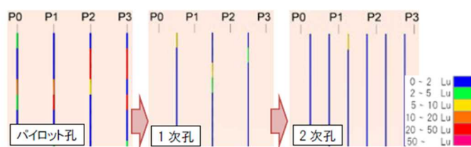
(d)カーテングラウチング改良状況
