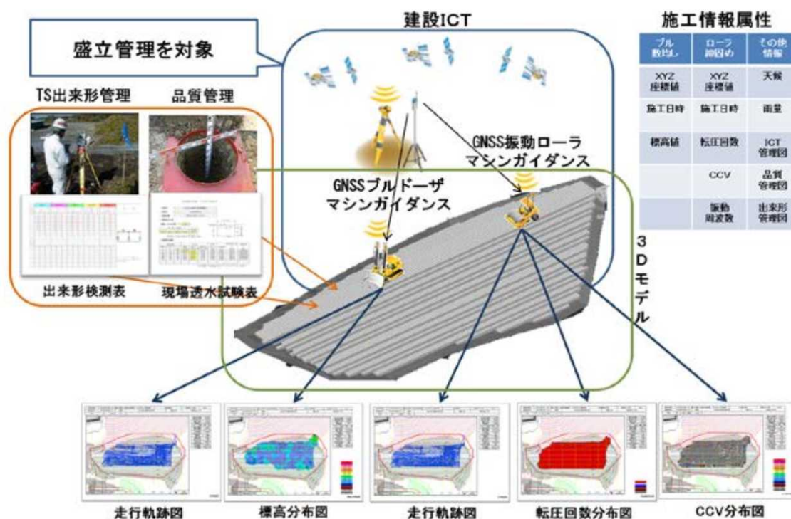
図 12 建設 ICT と CIM の一元化のイメージ
