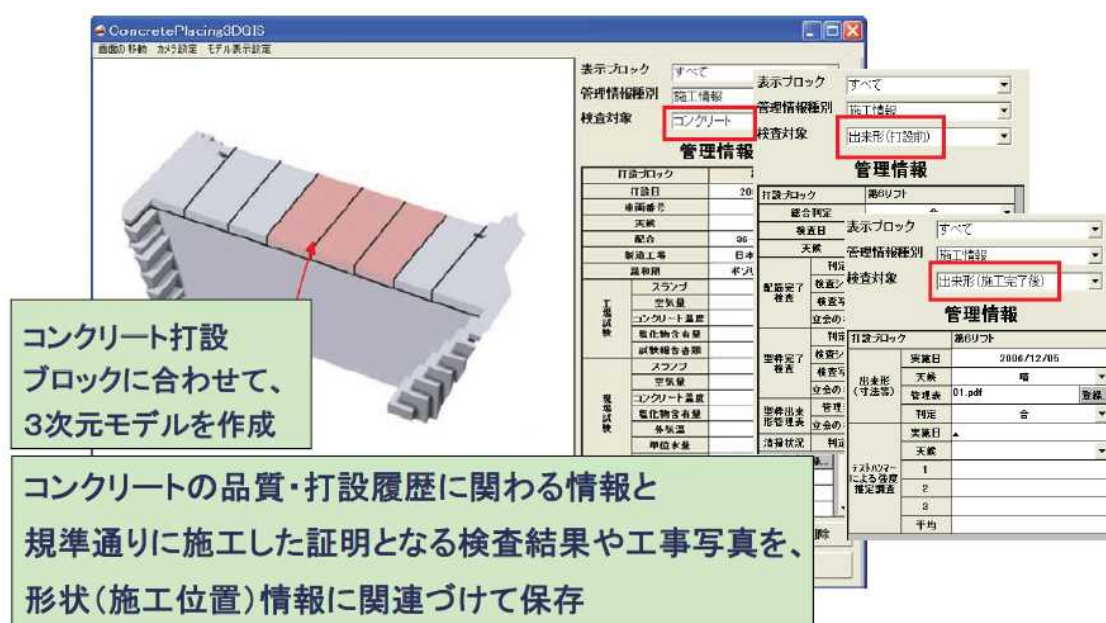
図 11 ダム CIM モデルへの施工情報の付与の例
