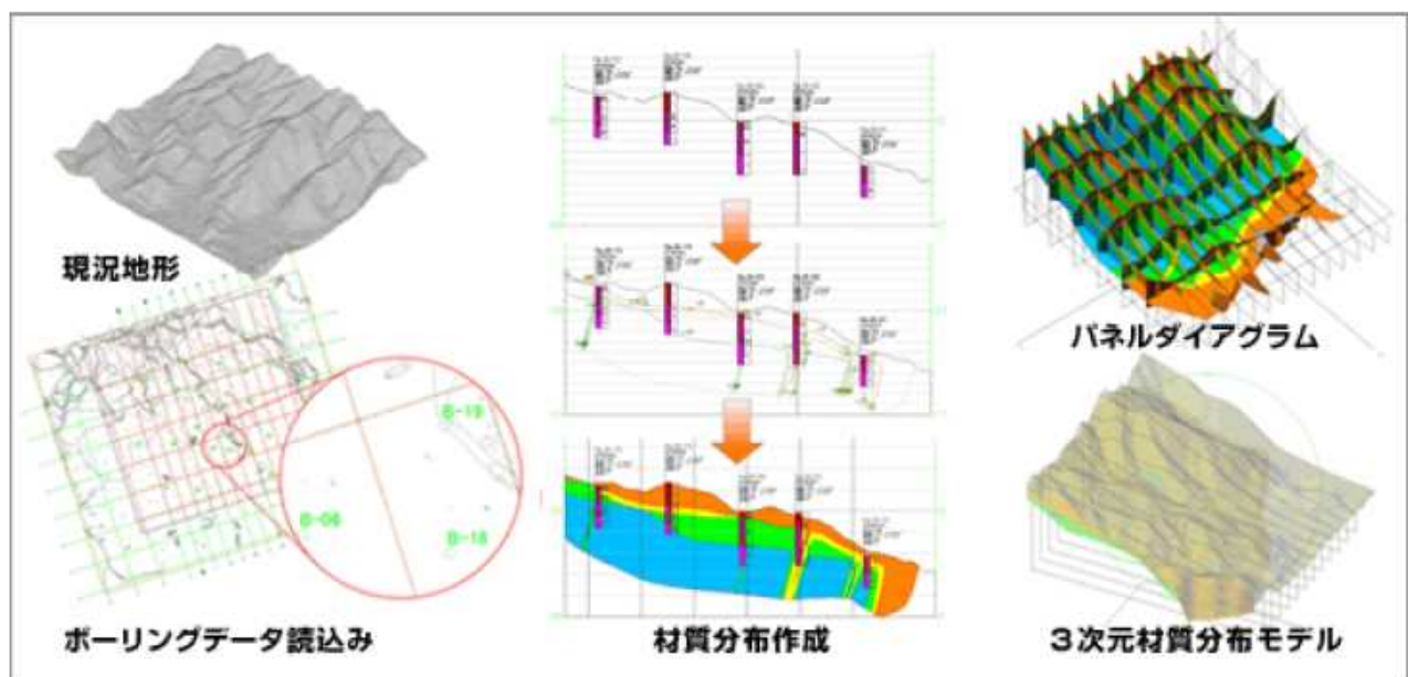
図 14 原石山の掘削による数量算出例①
