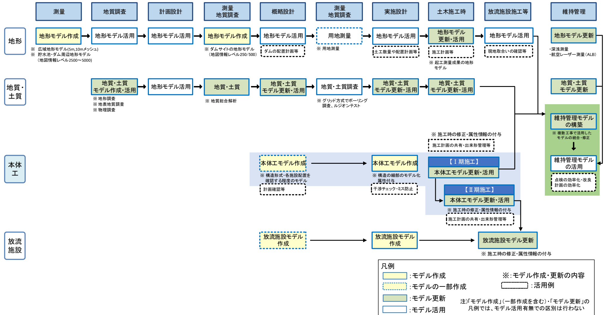
図 2 ダムにおける CIM モデルの作成、更新及び活用の流れの例
