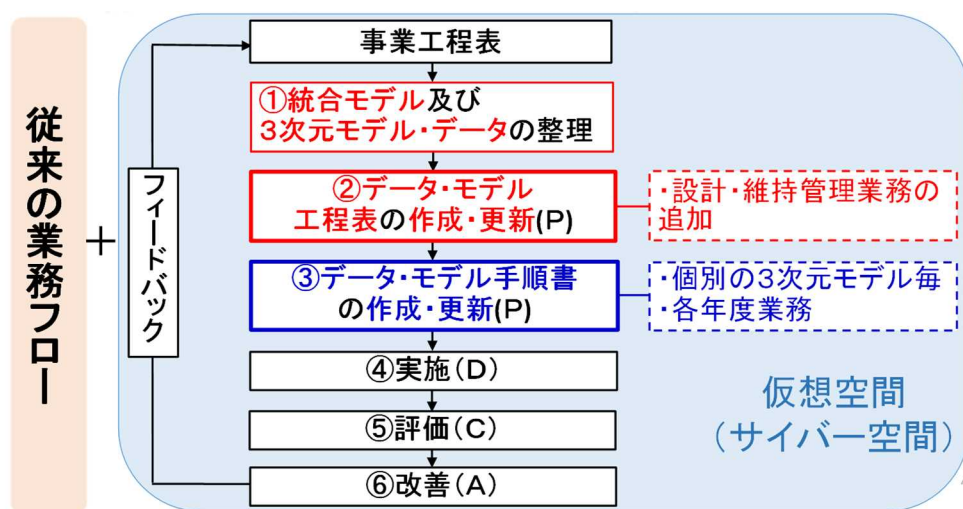
図 28 統合モデルを用いたダムマネジメントの概略フロー
