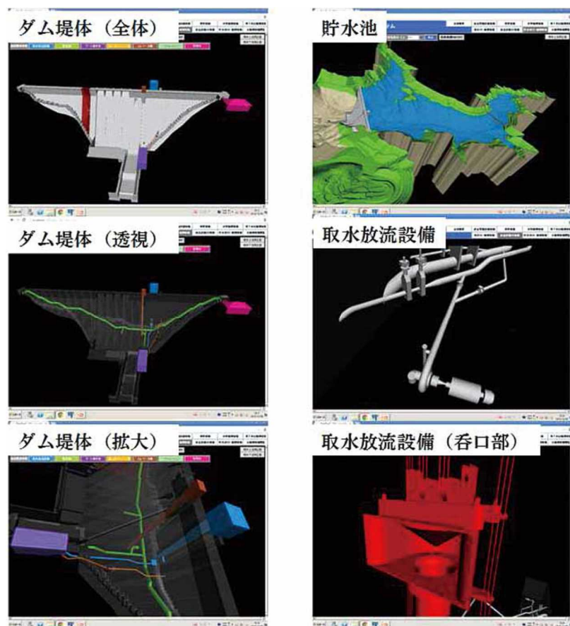
図 7 構造物モデルイメージ（大山ダムの例）
