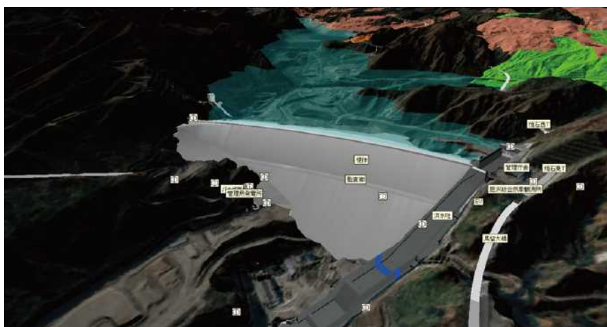
図 3 ダムの CIM モデル
