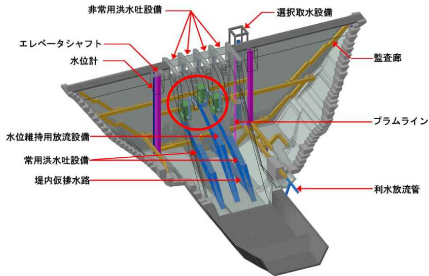
図 6 構造物モデルイメージ（ハッ場ダムの場合）
