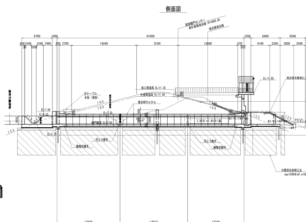
(b)3DA 面図への寸法、注記等の付与例
