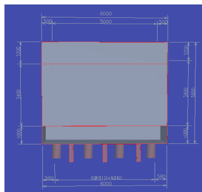
(b) 3DA 面図への寸法、注記等の付与例
