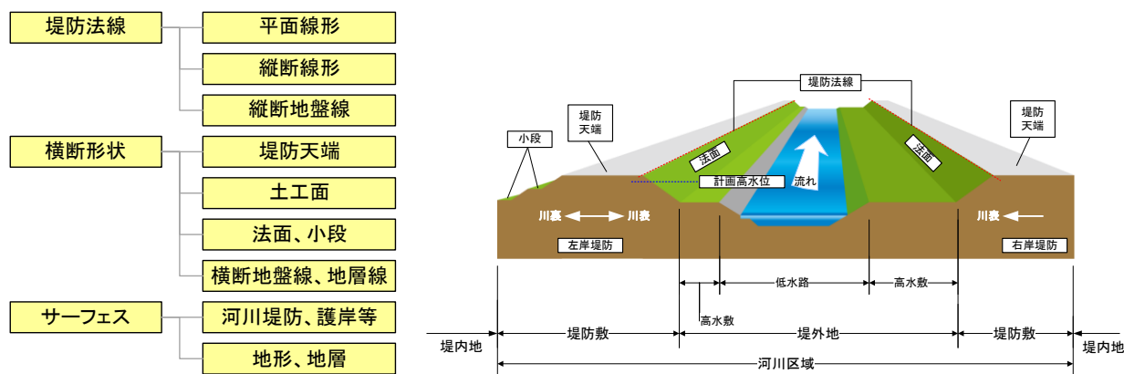
図 4-3 河川分野で対象とする要素とイメージ図
