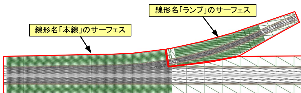
図 5-10 複数線形がある場合
