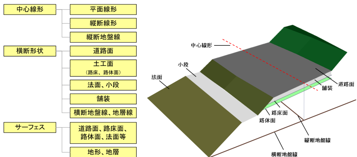
図 4-2 道路分野で対象とする要素とイメージ図
