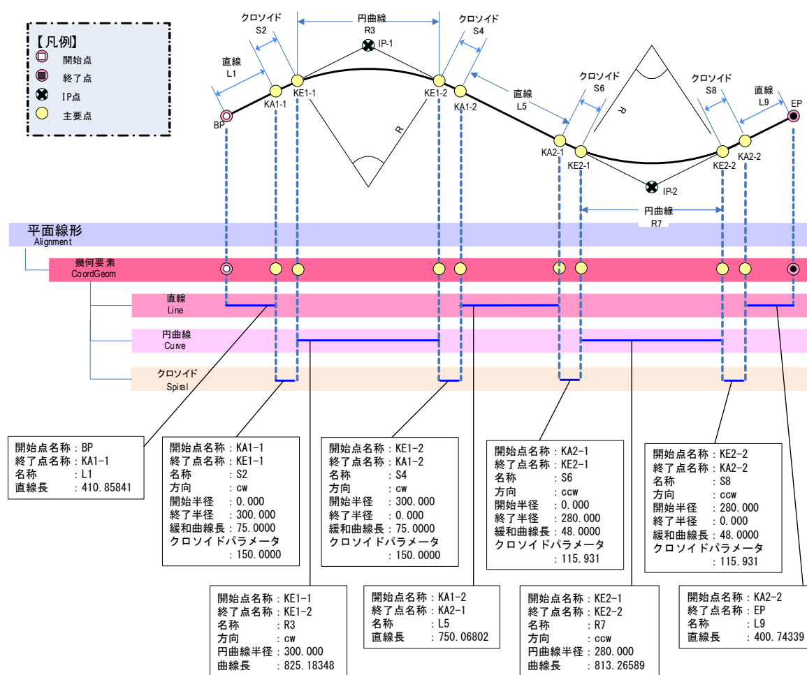
図 4-4 幾何要素の記述（例）
