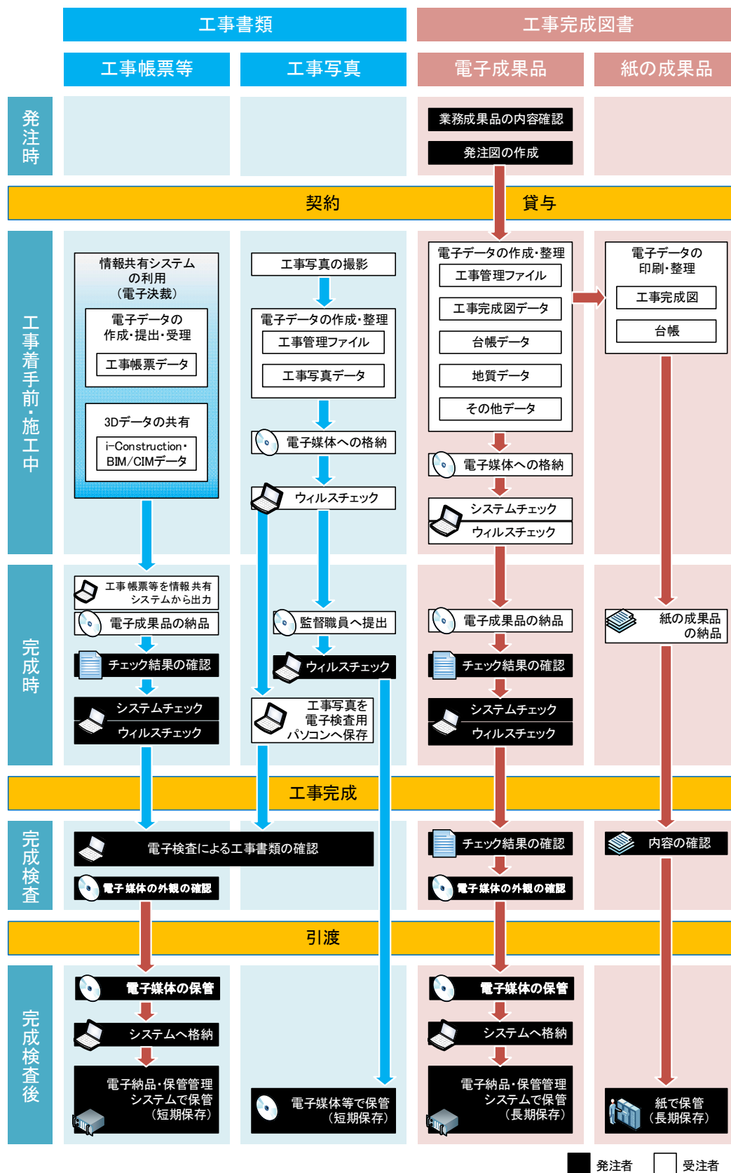
図 18 電子納品・電子検査の流れ（電子媒体で納品する場合）
