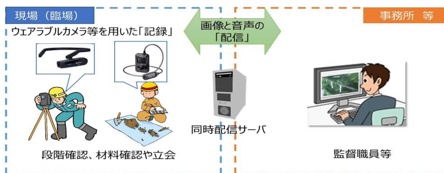
図 11 機器構成（例）
