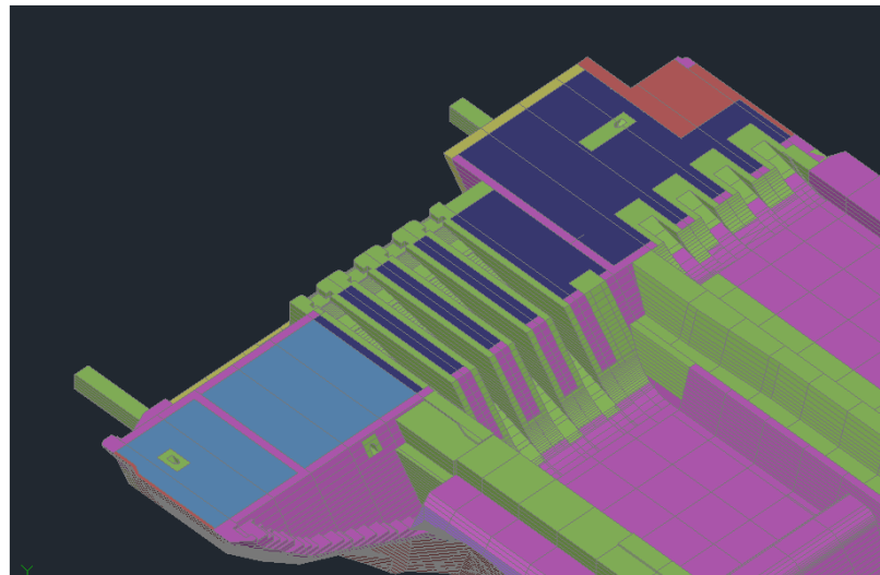
堤体スライス図
