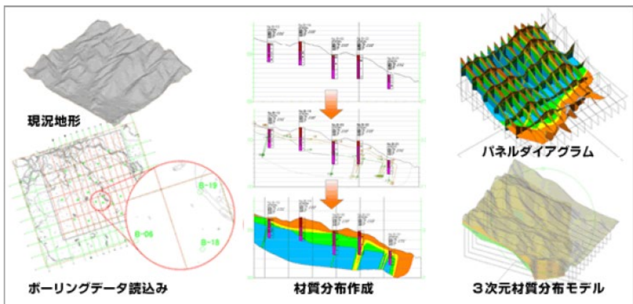
図 19 原石山の掘削による数量算出例①
