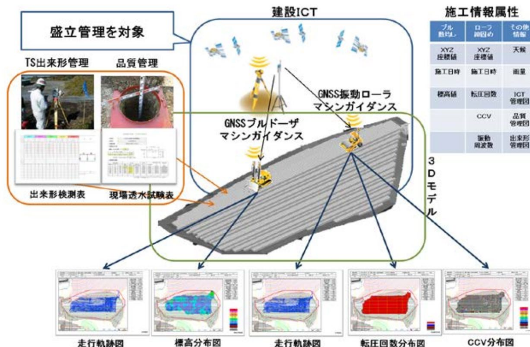
図 17 建設 ICT と CIM の一元化のイメージ
