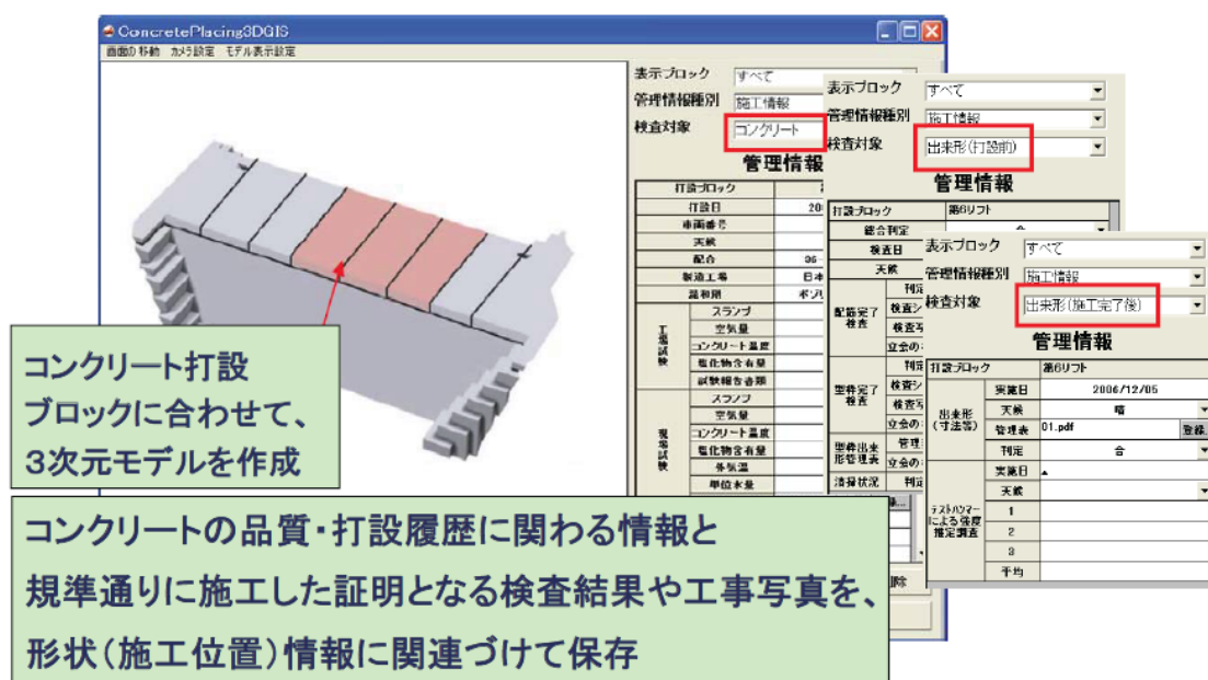
図 16 ダム BIM/CIM モデルへの施工情報の付与の例
