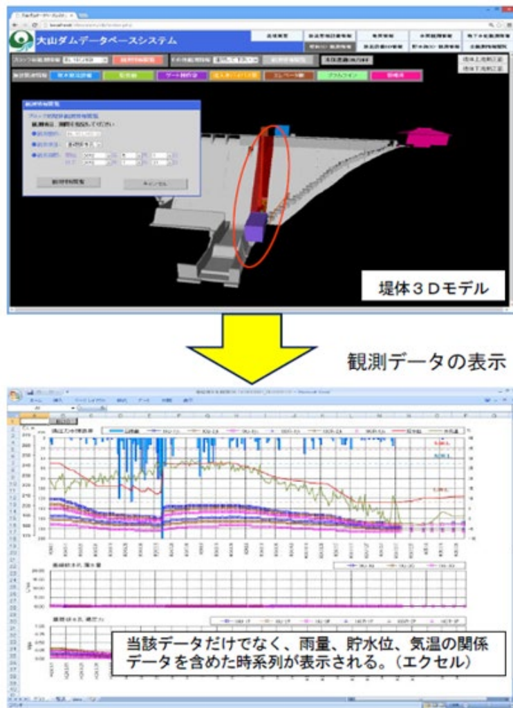
図 30 地下水位情報（大山ダムの事例）
