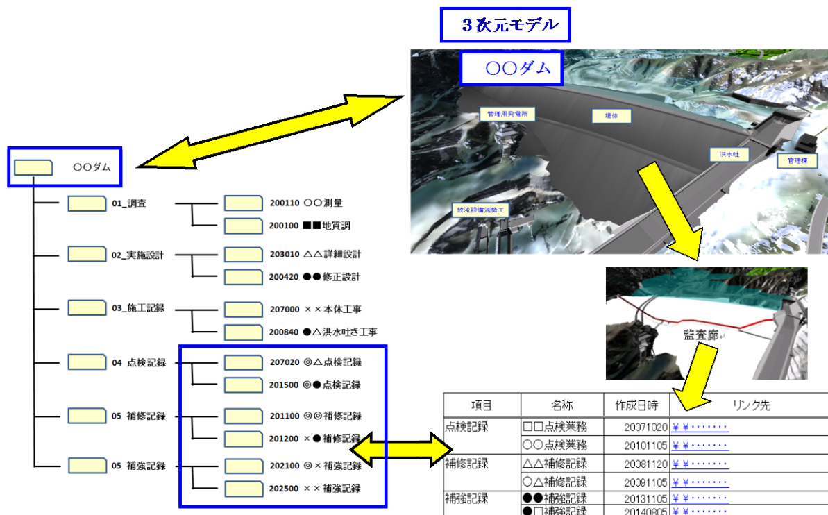
図 27 事例 BIM/CIM モデル作成指針 (データ構造) (検討案)
