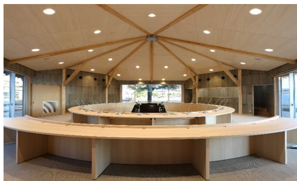
海上保安大学校 国際交流センター（広島県呉市）：国際講義棟（木造 軸組構法）
