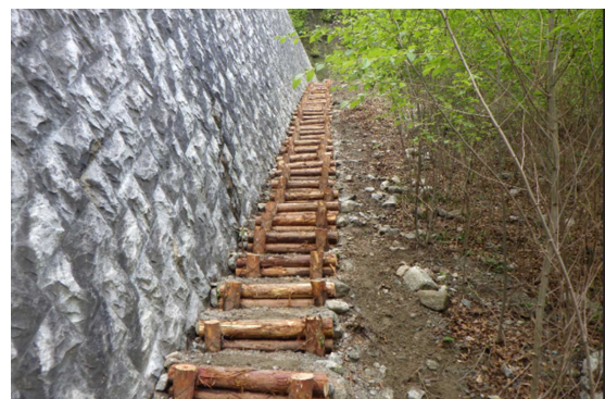
釜無川水系小武川（山梨県韮崎市） 『階段工』
