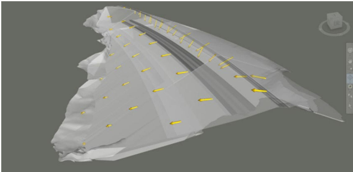
図 5-9 GPS 観測装置データによるダム堤体変位可視化例（胆沢ダム CIM モデル）
