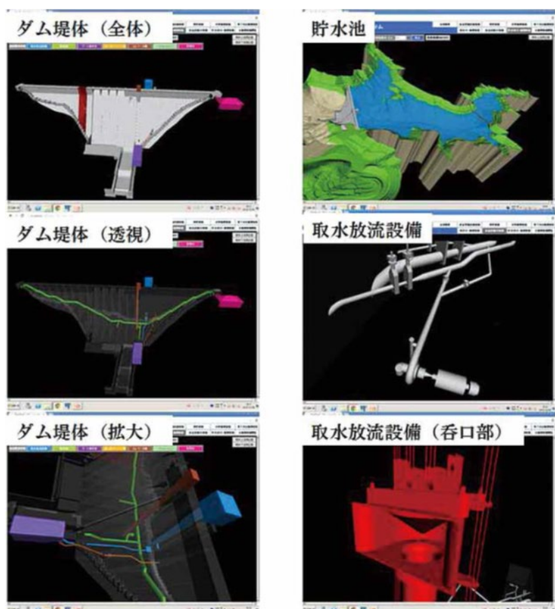
図 3-7 構造物モデルイメージ (大山ダムの例)
