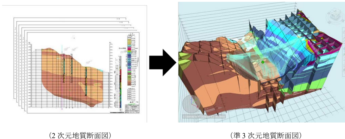
図 3-5 地質・土質モデルイメージ
