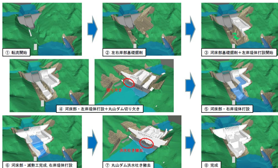
図 3-14 施工ステップ確認において活用する BIM/CIM モデルの例
