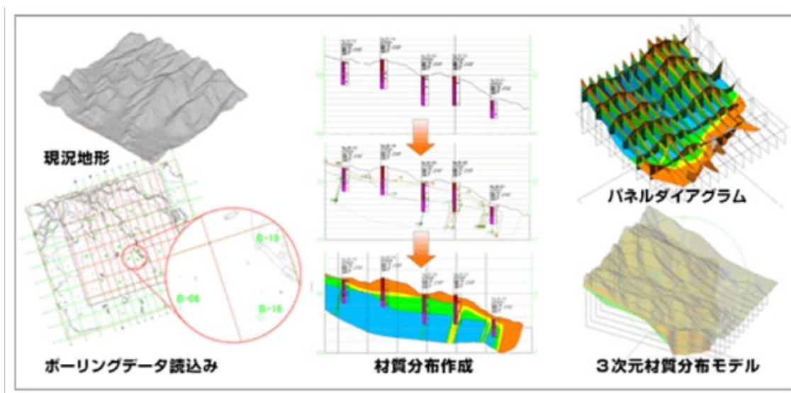
図 4-4 原石山の掘削による数量算出例①
