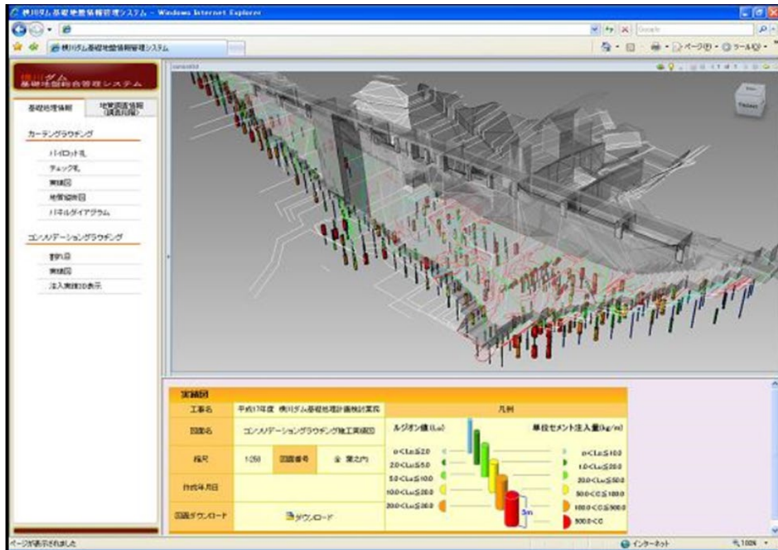
図 5-11 ダム基礎地盤コンソリデーショングラウチングの3次元可視化
