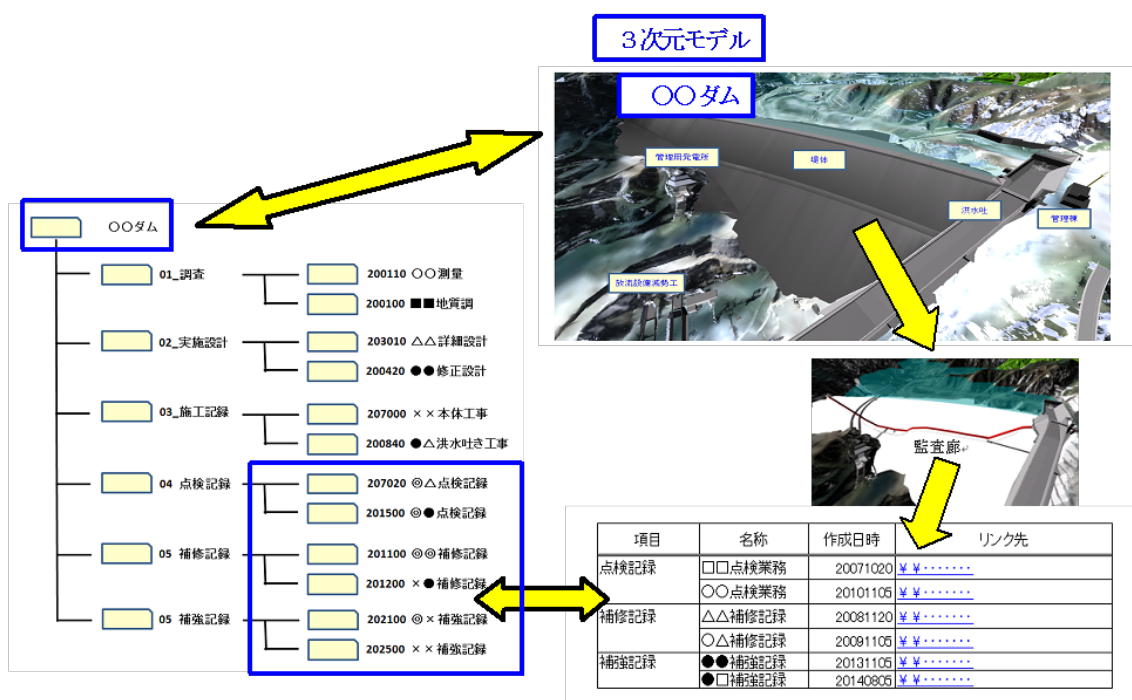
図 5-7 事例 BIM/CIM モデル作成指針（データ構造）（検討案）
