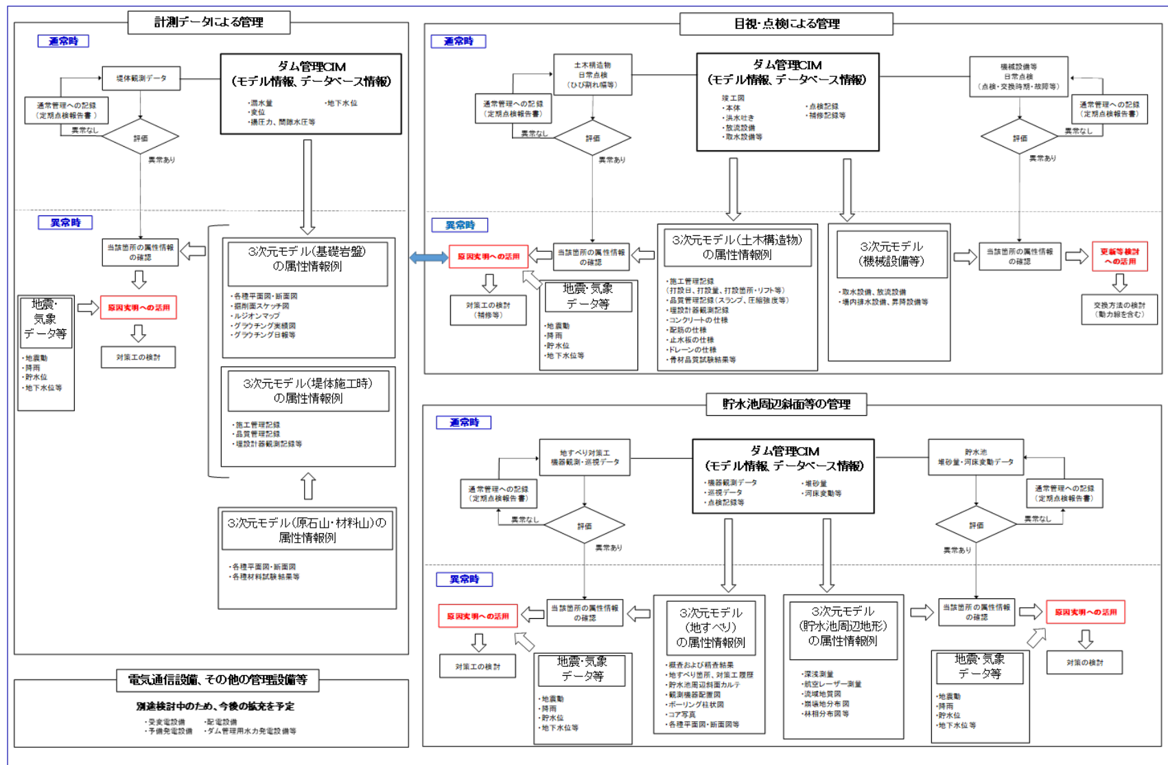
図 5-8 ダム管理 BIM/CIM の活用フロー (案)
