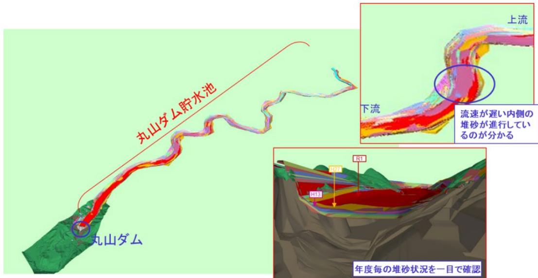
図 5-12 ダム統合モデルの堆砂データの可視化
