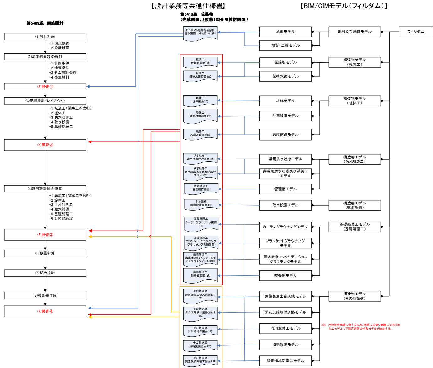
図 3-2 フィルダムにおける BIM/CIM モデルの作成、更新及び活用の流れの例
