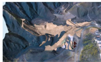
基礎掘削完了・仮設備配置
