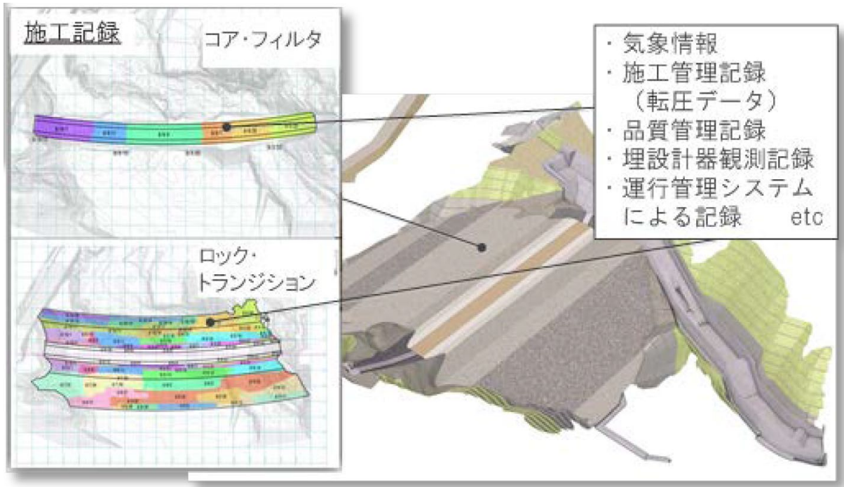
図 4-3 盛土材料・品質情報の管理
