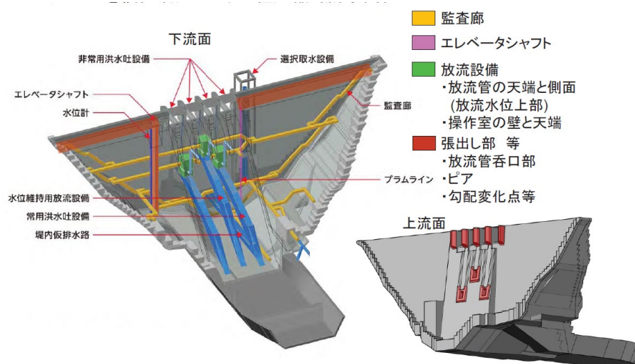
図 3-6 構造物モデルイメージ (ハッ場ダムの例)
