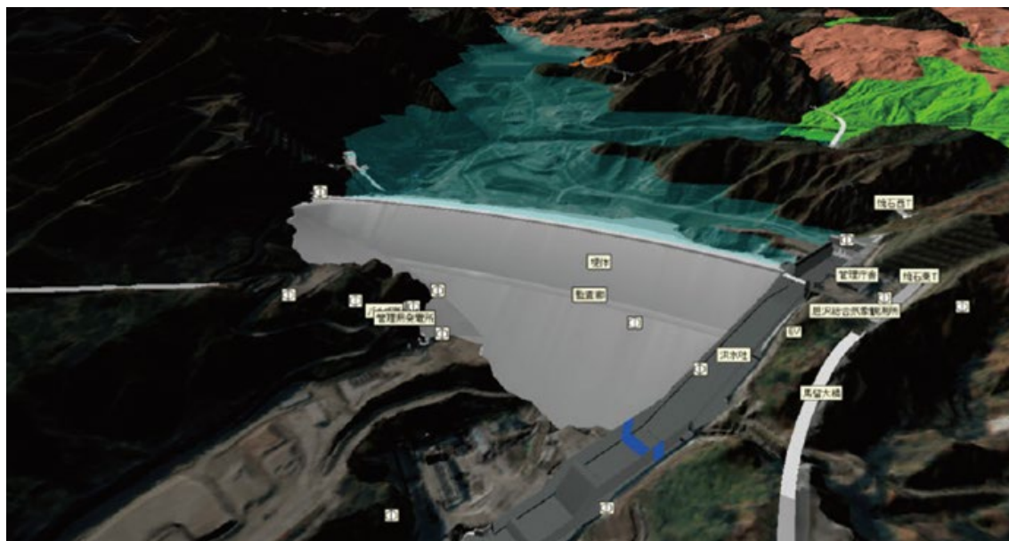
図 3-3 ダムの BIM/CIM モデル
