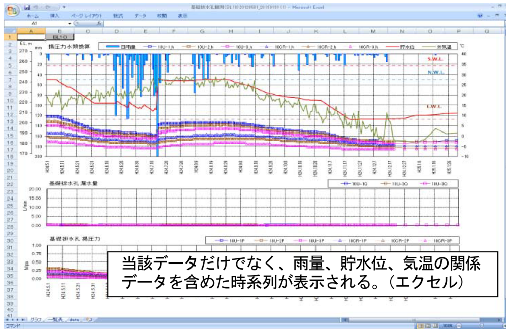
図 5-10 地下水位情報（大山ダムの事例）
