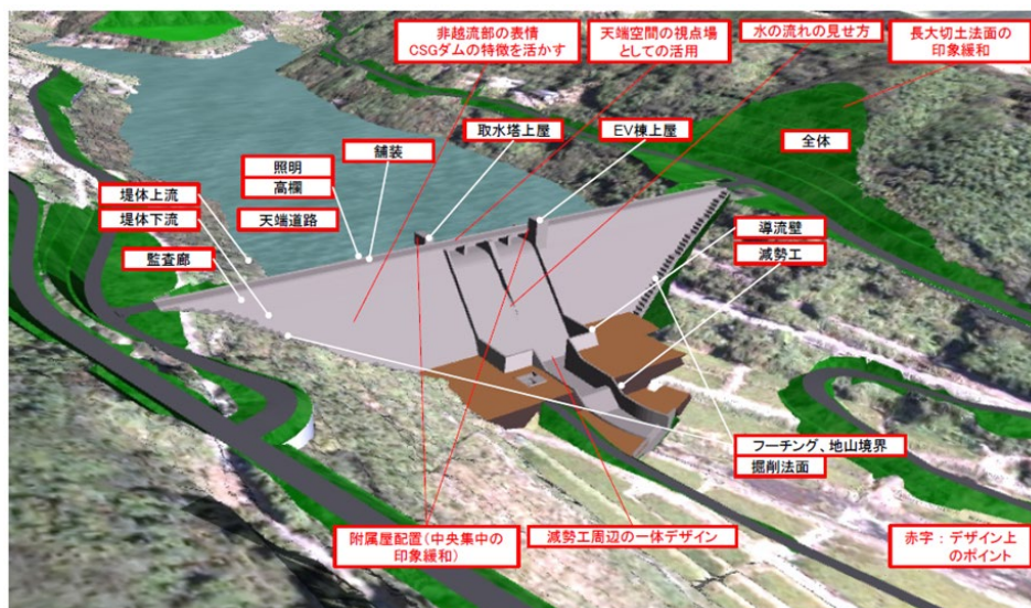
構造物のデザイン検討図
