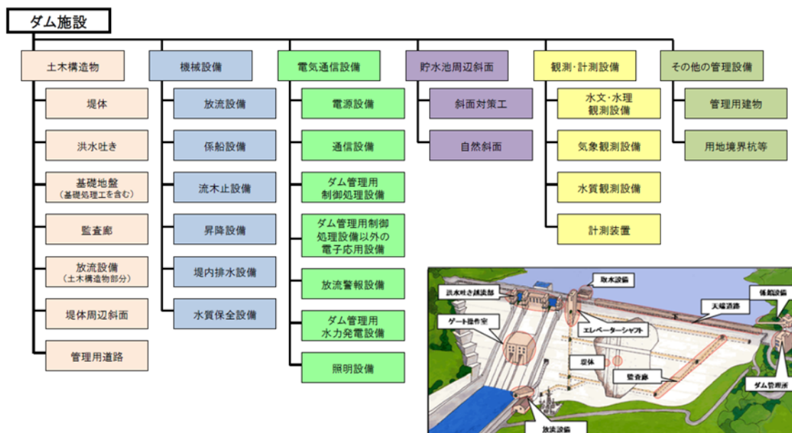
図 5-2 ダム施設の構成
