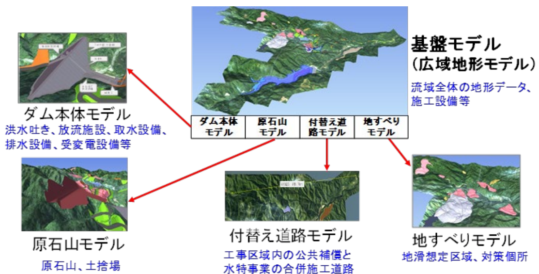
図 5-13 ダム統合モデルの例
