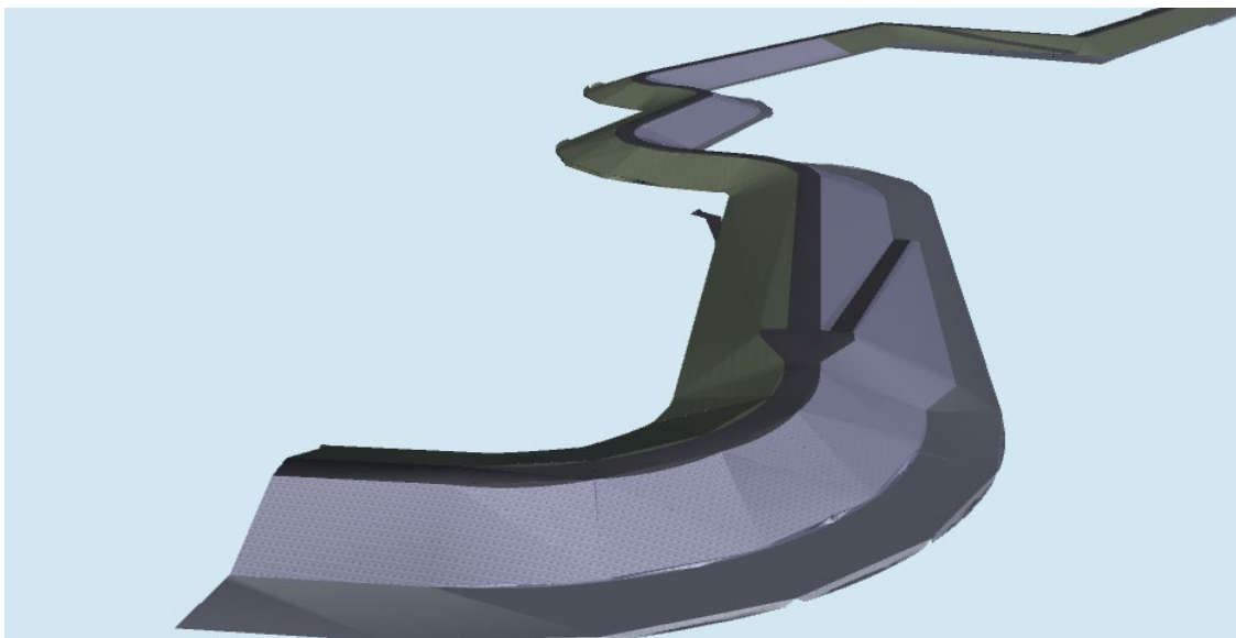
図 2-6 土工形状モデルの例
