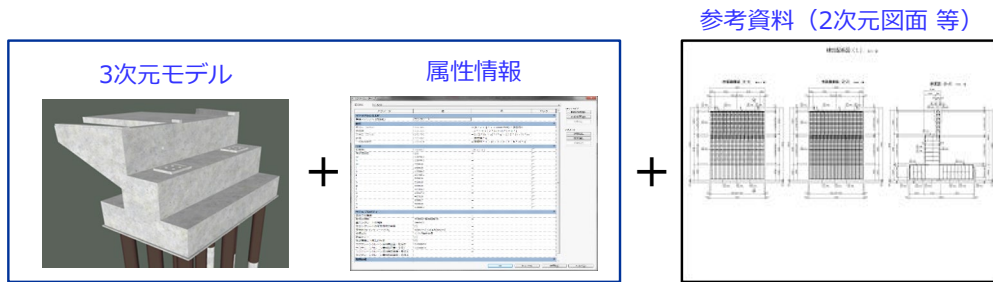
図 2-7 構造物モデルの例
