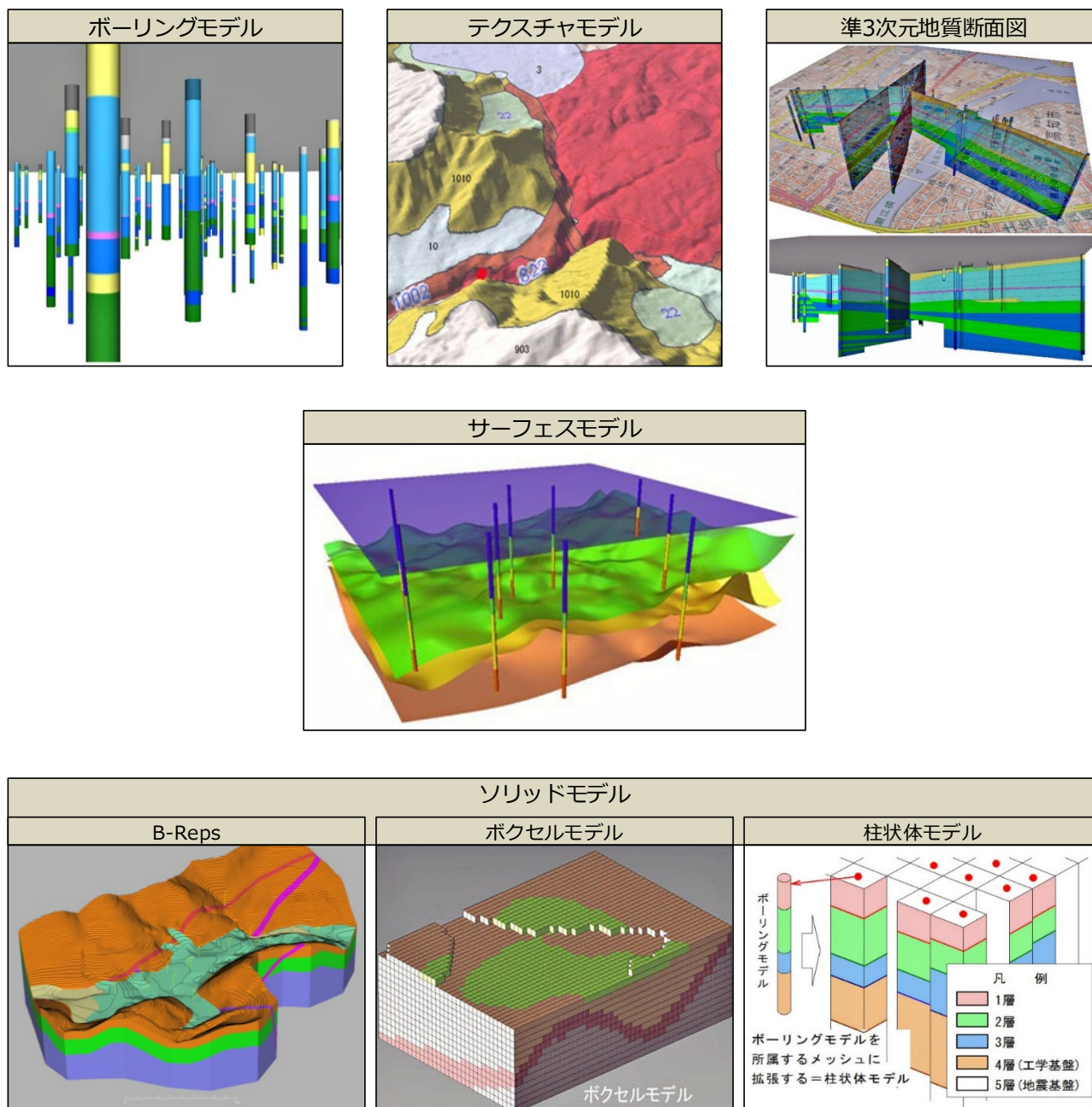
図 2-4 地質・土質モデルの例
