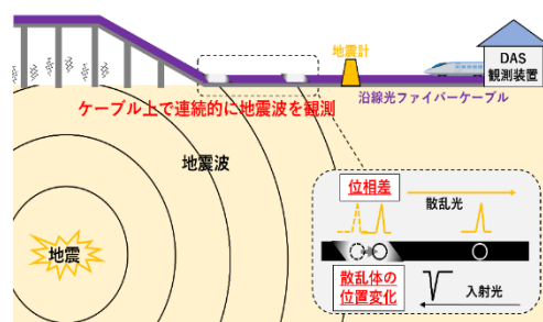
鉄道沿線でのDAS地震観測イメージ
