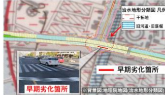
舗装状態や修繕履歴等の見える化 要調査箇所の抽出、調査の実施
