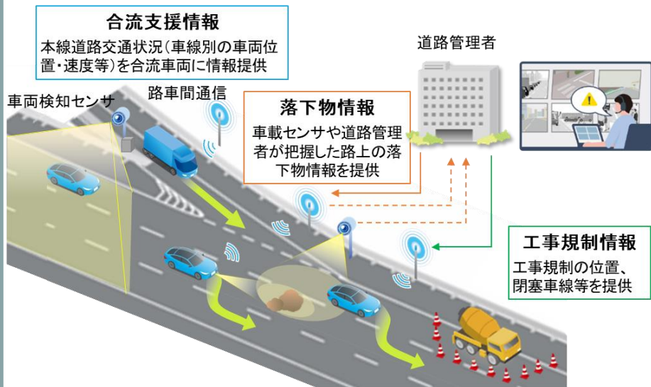
高速道路における自動運転トラックの実現に向けた実証実験の実施イメージ
