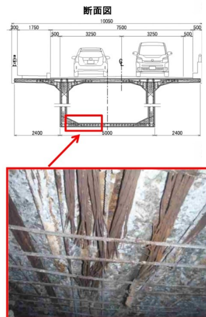
■現在の妙高大橋の損傷状況
