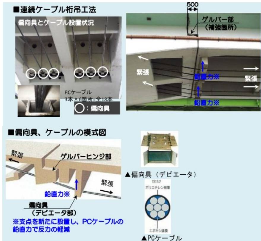
図-2-14-1 連続ケーブル桁吊工法
