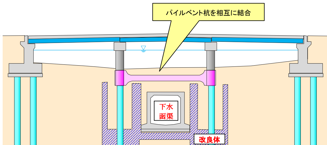
図-2-10-1 高知橋耐震補強側面図
