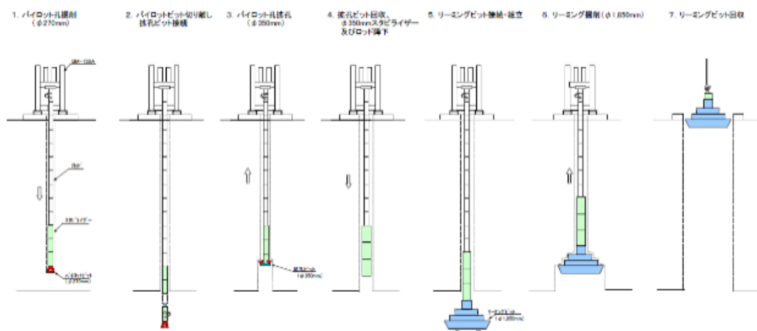
図-2-17-2 レイズボーリング工法による立坑掘削模式図
