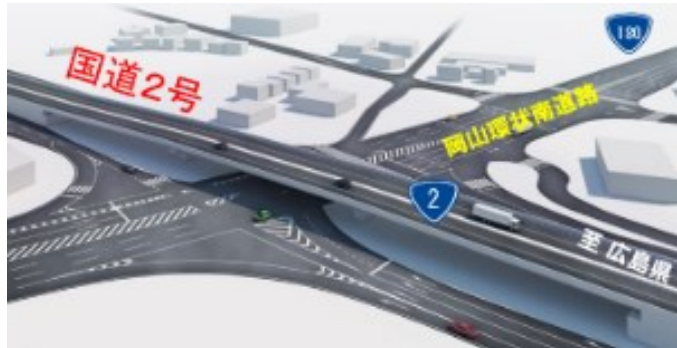
図-2-6-1 大樋橋西高架橋
