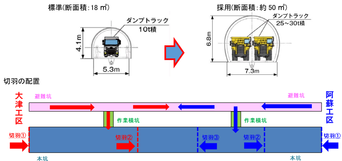
図-2-2-1 二重峠トンネルの施工
