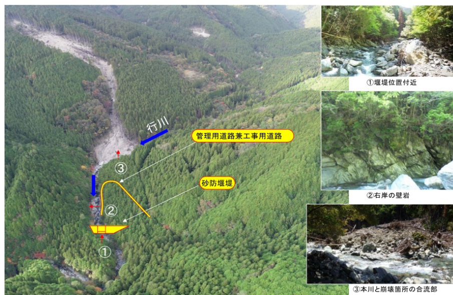
写真-2-20-1 行川本川砂防堰堤工事
