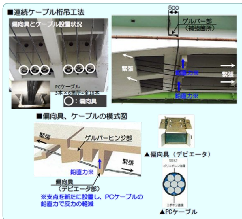
図 参 13-1 国道3号千歳橋補修工事
