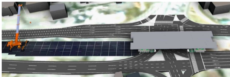
図-2-6-2 多軸式特殊台車を用いた大ブロック架設
