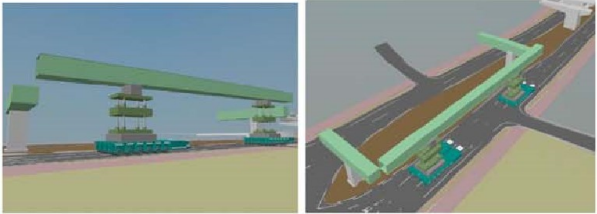
図-2-7-2 BIM/CIM を用いた架設計画検討
