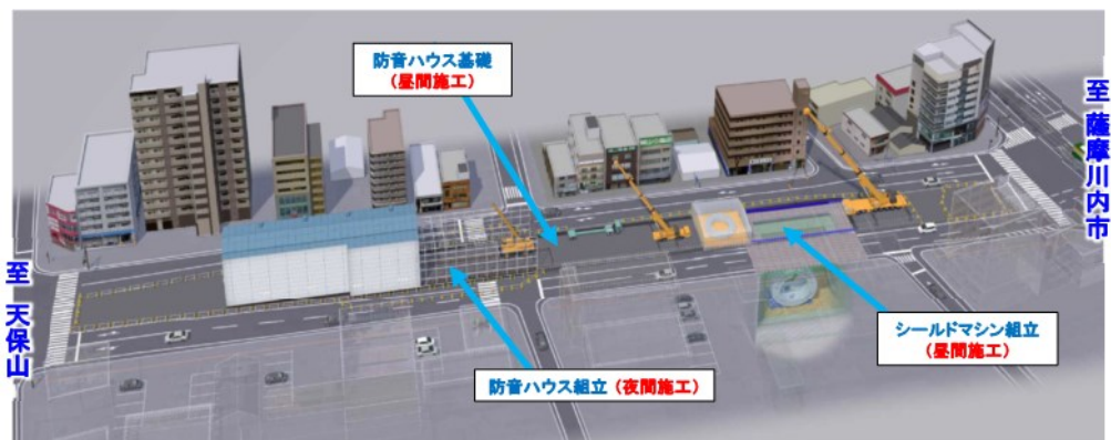
図-2-11-2 BIM/CIM を用いた地元説明資料
