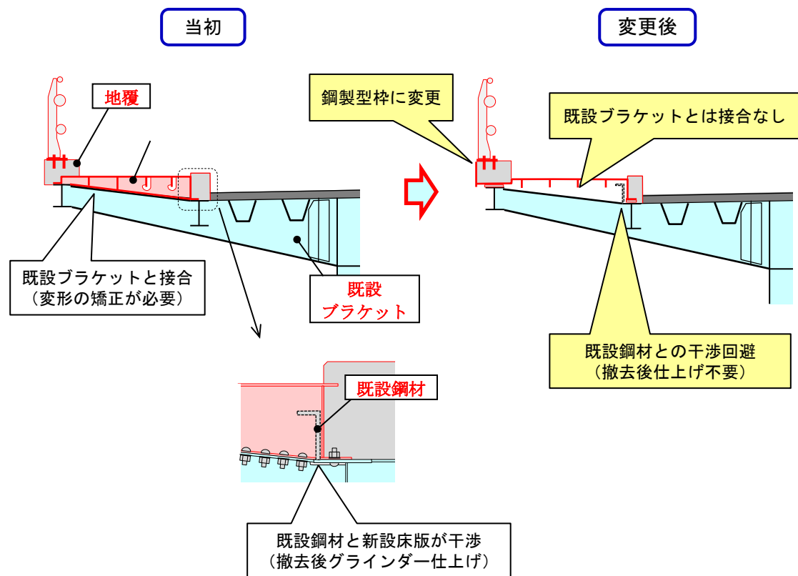
図-2-12-2 新設床版支持方法の変更
