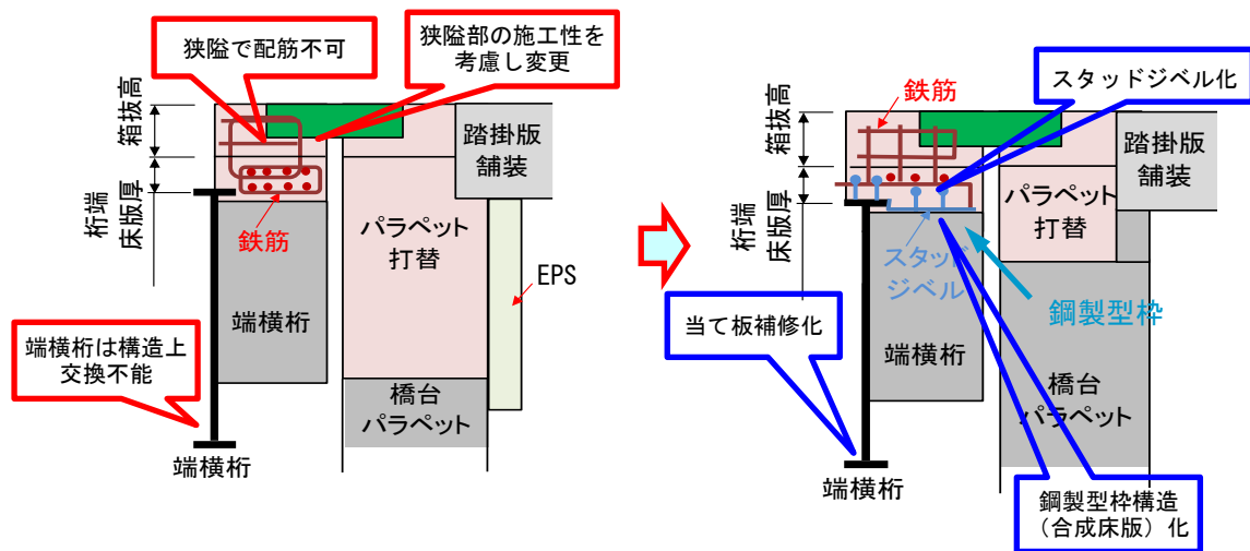
図-2-4-1 犀川大橋伸縮装置周辺部の構造変更
