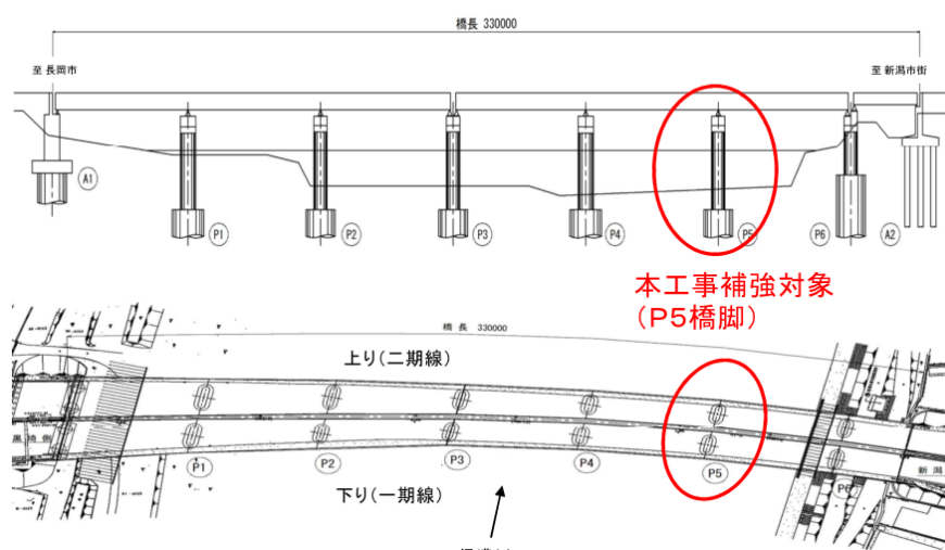
図-2-18-1 新潟大橋
