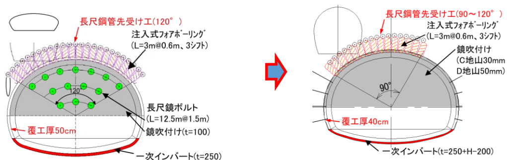
図-2-5-2 城山トンネルの施工
