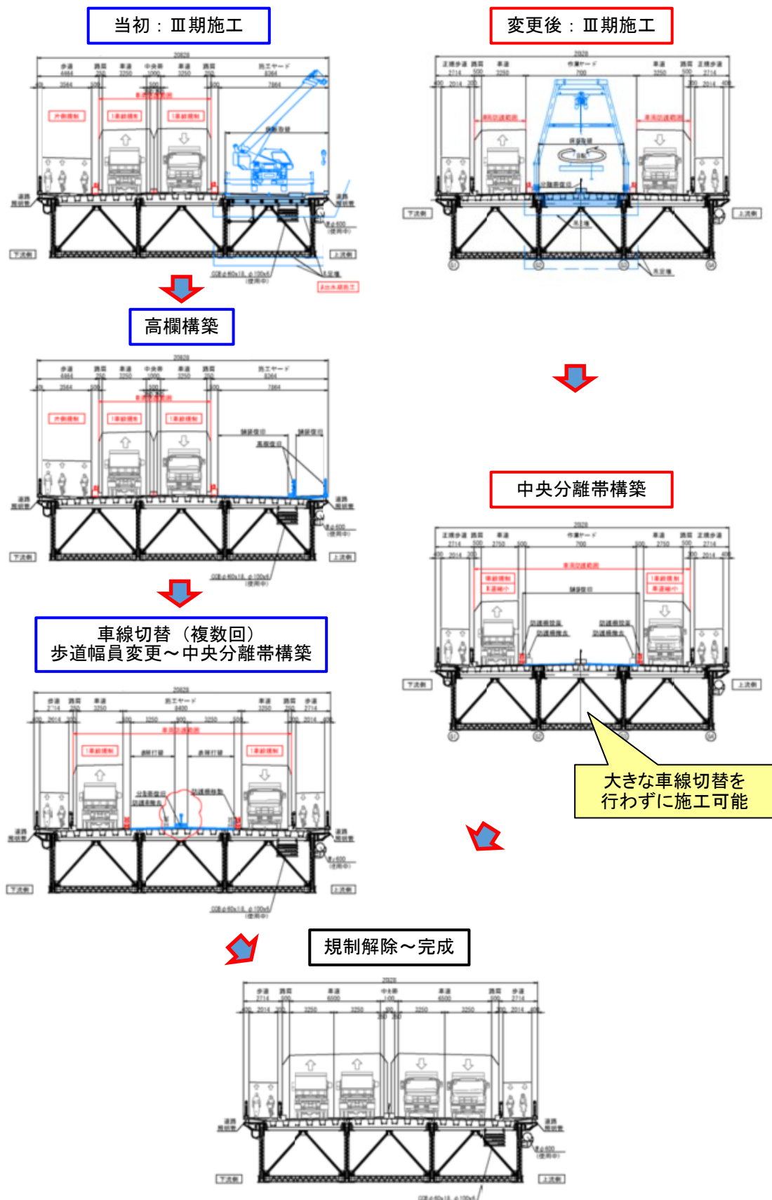
図-2-1-2 淀川大橋床版取替の車線切替の変更（Ⅲ期以降の主要ステップを記載）
