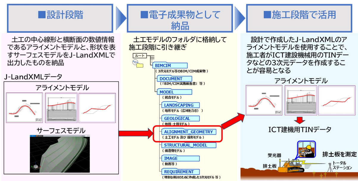
図 - 11 ICT 施工における BIM/CIM データの有効活用
