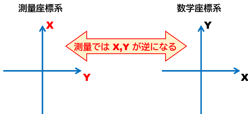
図 - 4 測量成果と数学座標のX軸Y軸の違い
