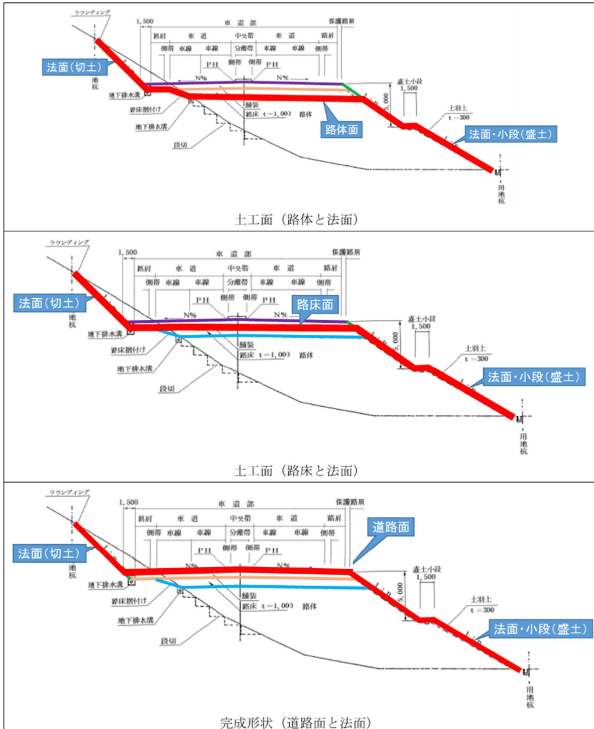
図 - 13 道路分野で ICT 施工に必要な断面
