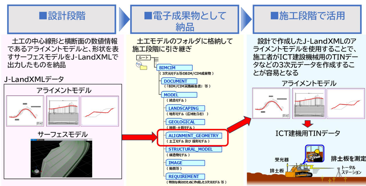
図 - 11 ICT 施工における BIM/CIM データの有効活用
