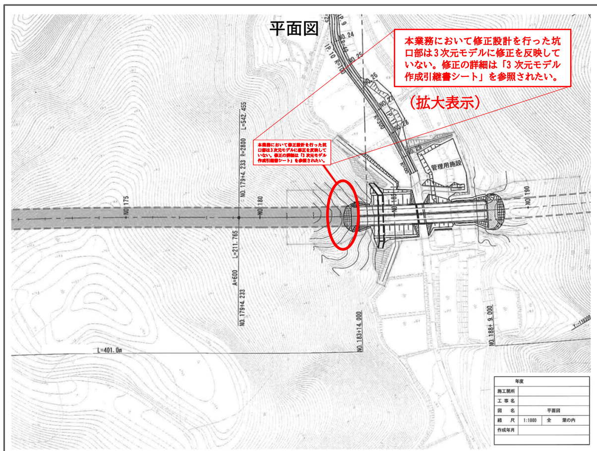
図 - 8 2次元図面への注釈記載例（トンネル修正設計）
