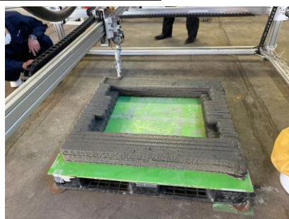
3Dプリンタで具現化（集水桝）
