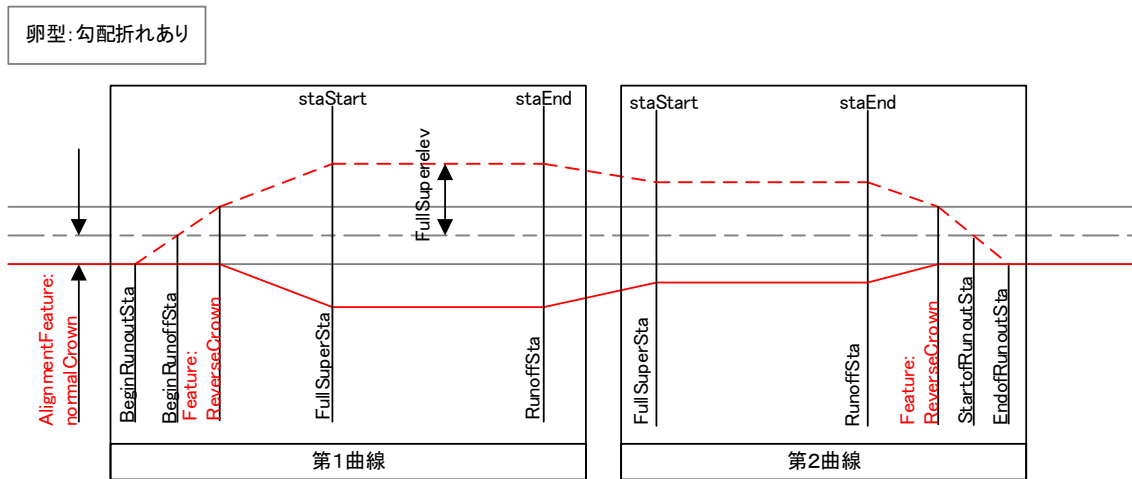
図 4-10 片勾配すりつけの例（卵型）
