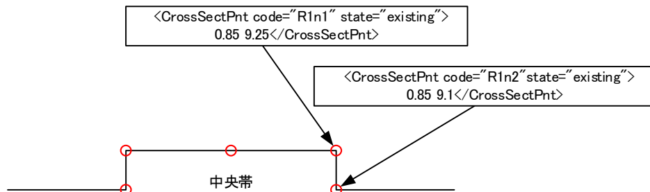
図 4-22 中央帯の作成方法
