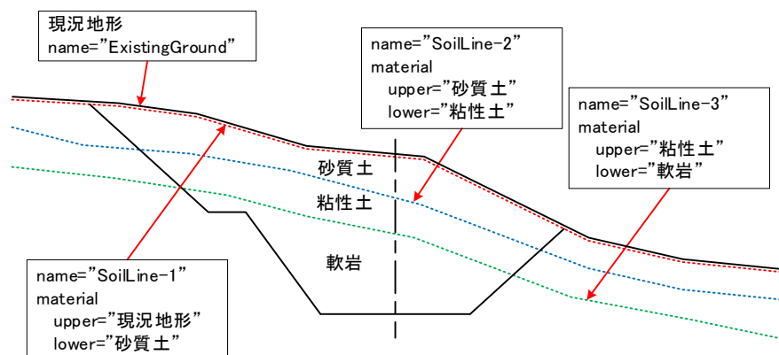
図 4-33 地形線を用いた地層表現例 (1)
