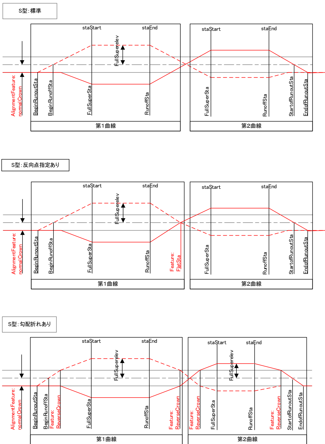
図 4-9 片勾配すりつけの例 (S 型)
