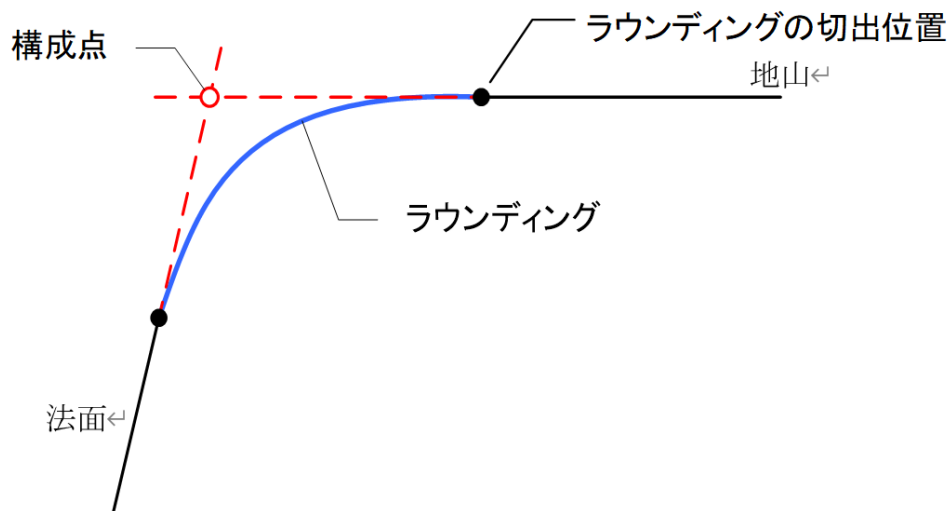
図 4-14 ラウンディングの定義方法
