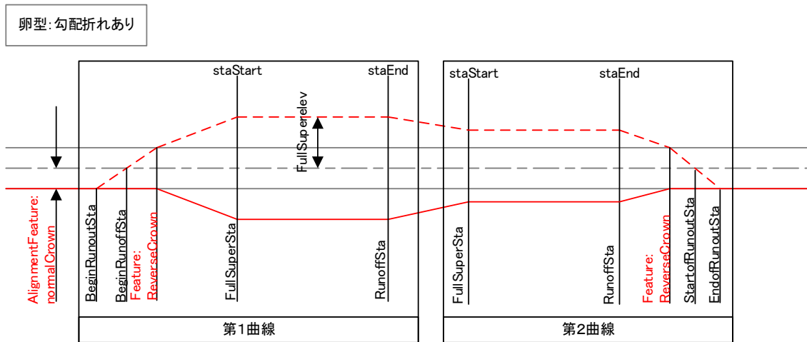
図 4-10 片勾配すりつけの例（卵型）
