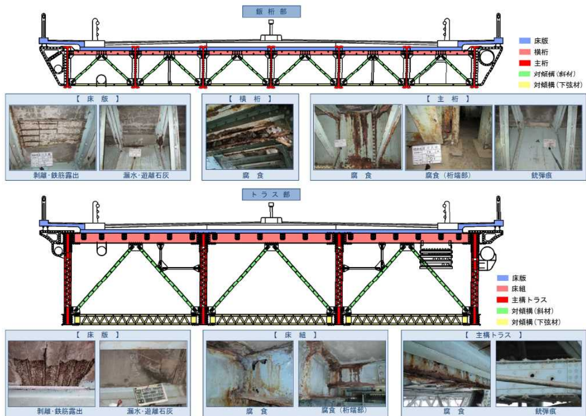
図 7-1-3 国道2号淀川大橋の損傷状況
