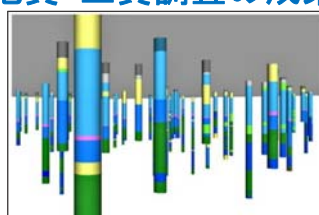
ボーリング柱状図
