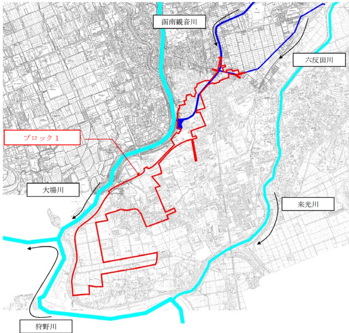
様式-1 氾濫ブロック分割図
