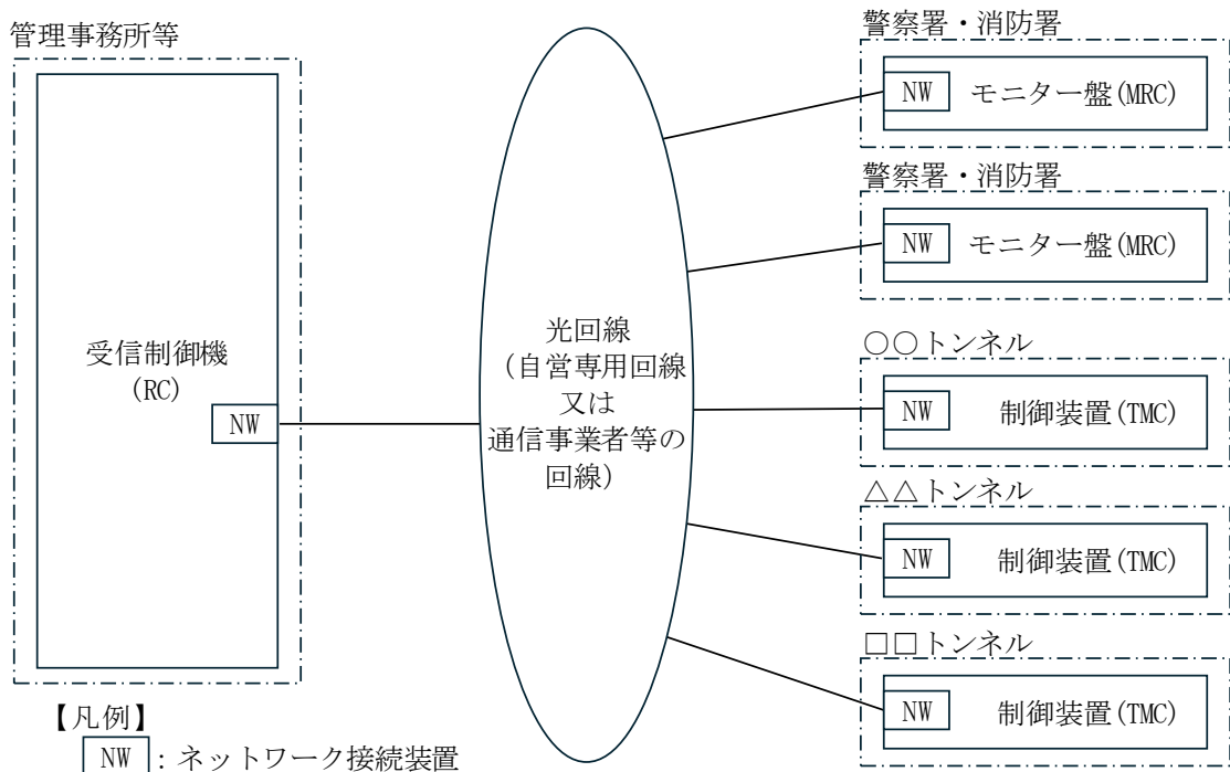
図 1-2 光回線でのシステム構成図
