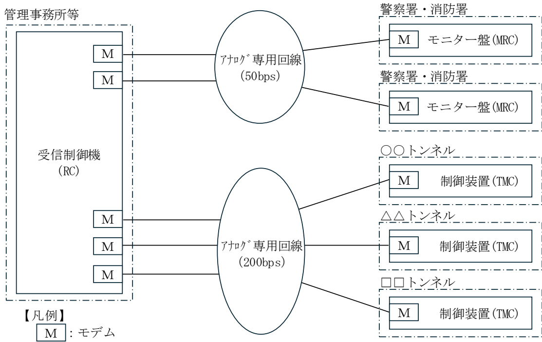
図 1-1 現行の専用線でのシステム構成図
