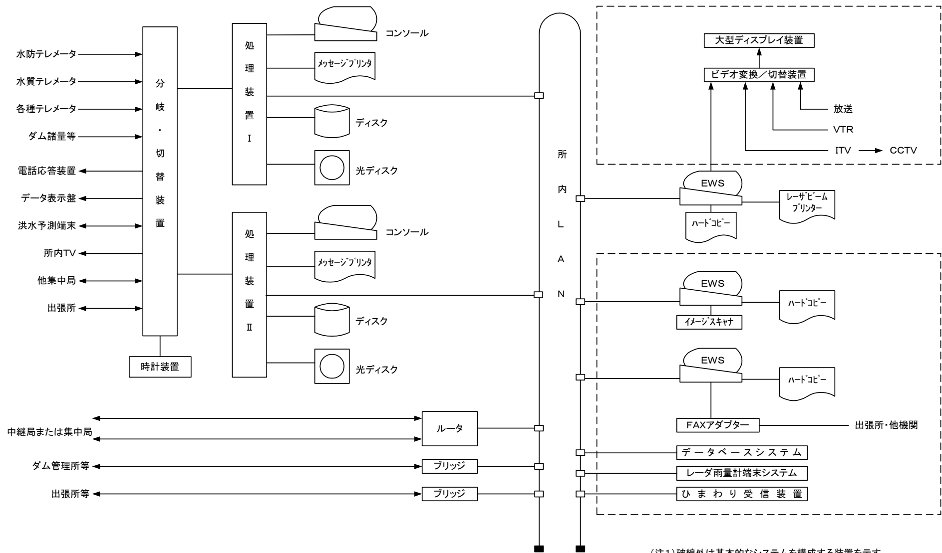
図16-1-2 河川情報システム(集中局システム二重化)のハードウェアシステム構成図
