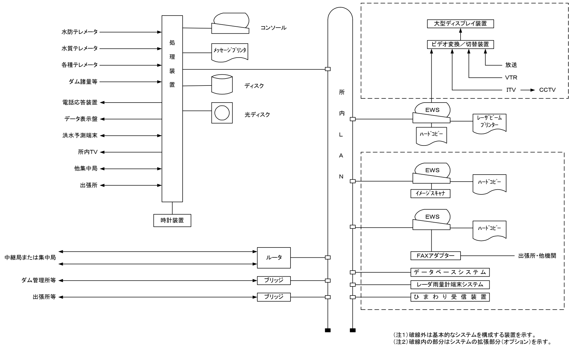
図16-1-1 河川情報システム(集中局システム)のハードウェアシステム構成図
