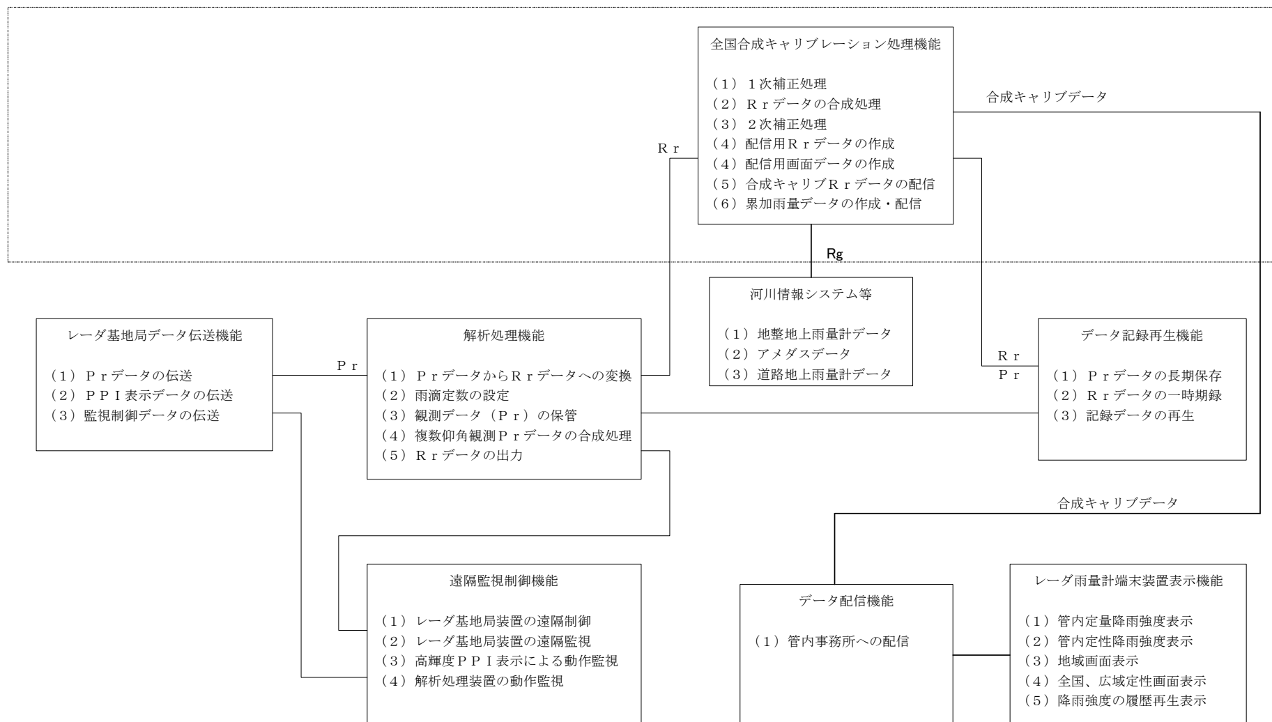
図16-4-2 解析処理局装置及び合成処理局装置の機能構成
