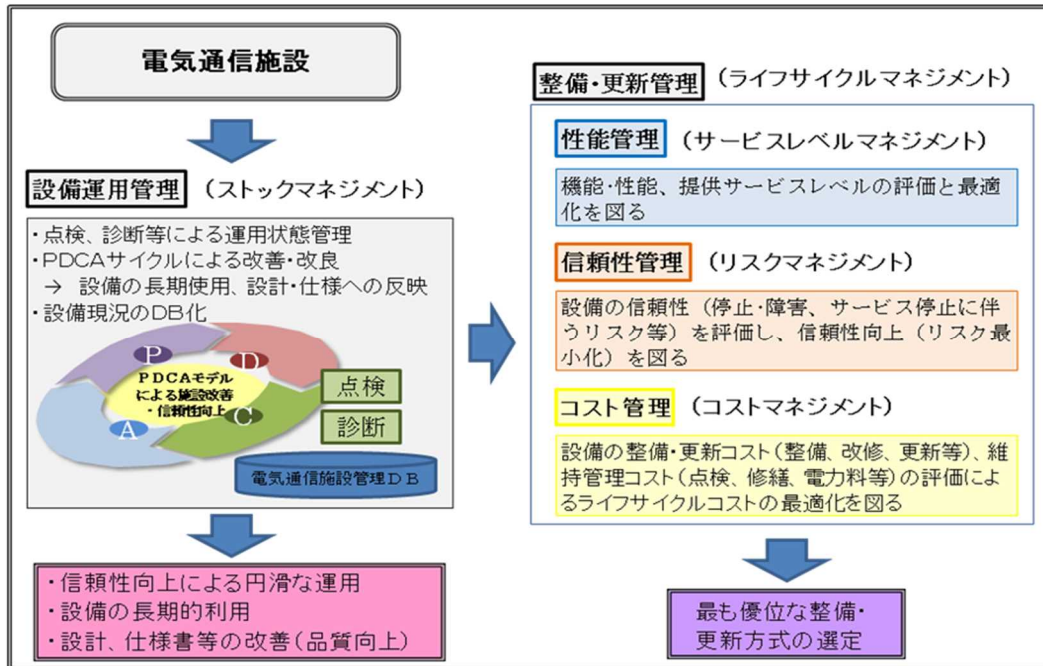
図-2 電気通信施設のアセットマネジメントの概念
