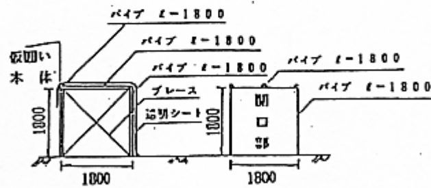
断面図
