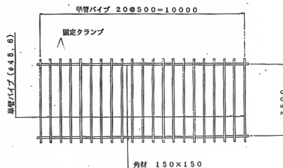
平面図 S=1/100
