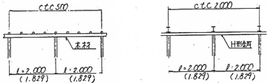
配 置 図
