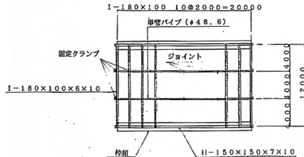
平面図 S=1/300
