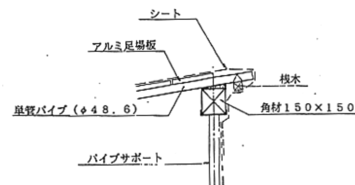
端部詳細図 S=1/20
