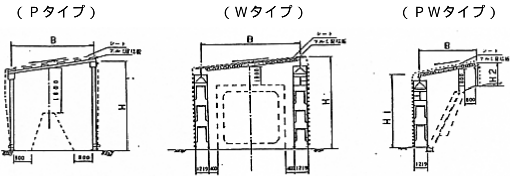
配置図
