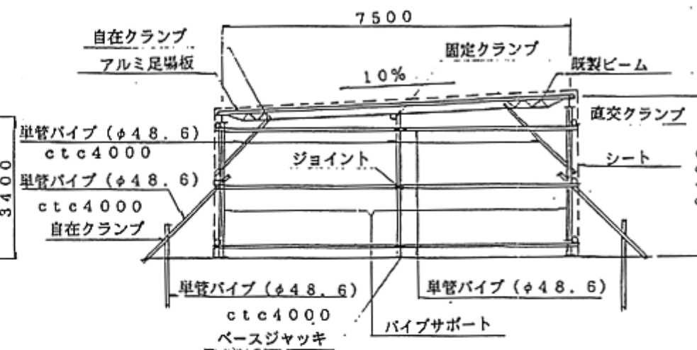
断面図 S=1/100
