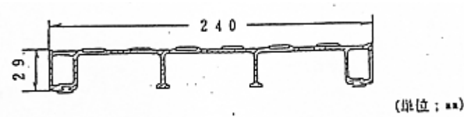
断面性能
