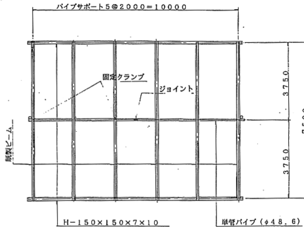
平面図 S=1/100
