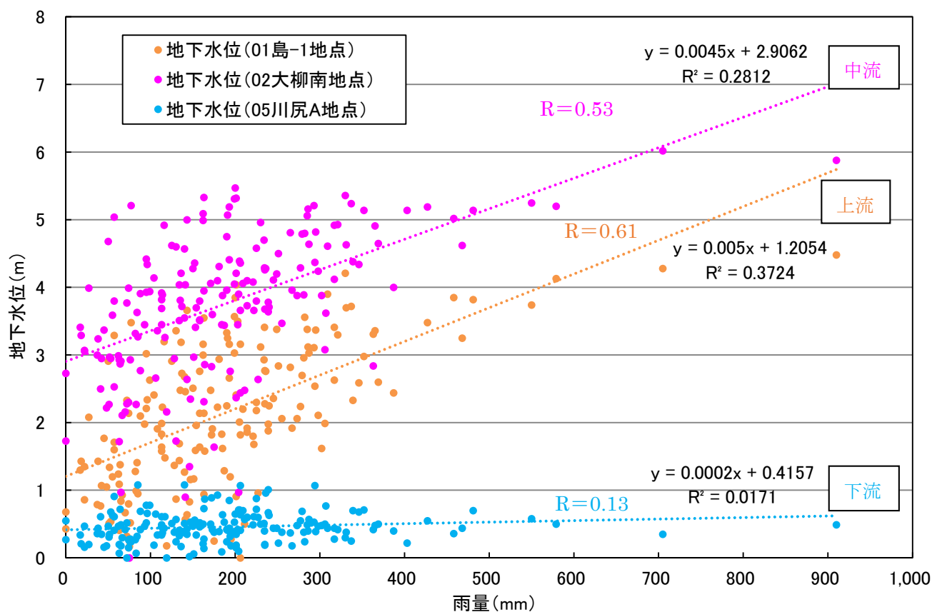
図 2.23 (2) 地下水位と島田観測所雨量の相関関係 (拡大図)
