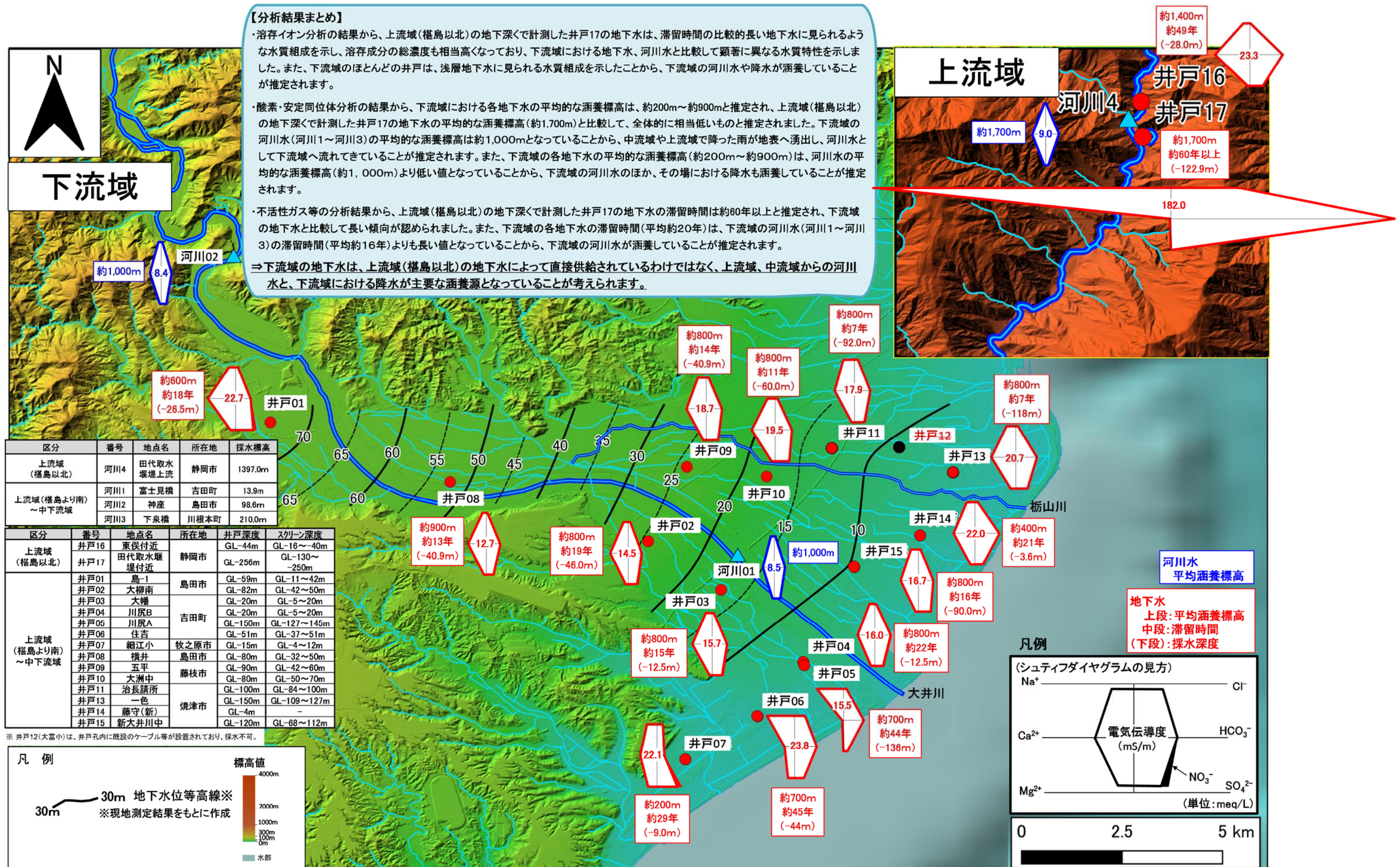
図 2.30 成分分析結果まとめ
