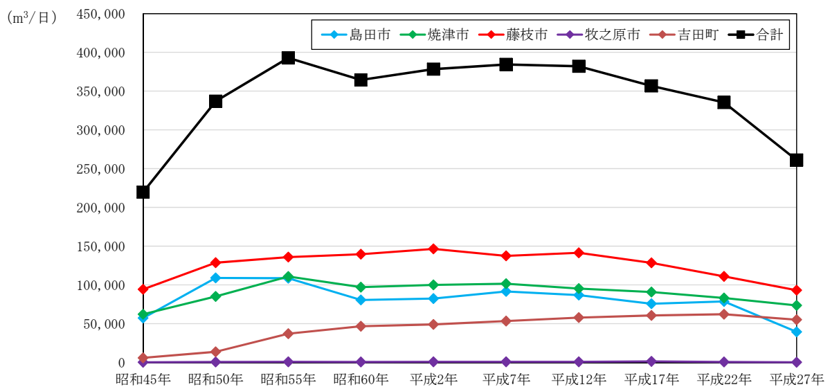
図 2.15 大井川下流域における地下水の利用状況
