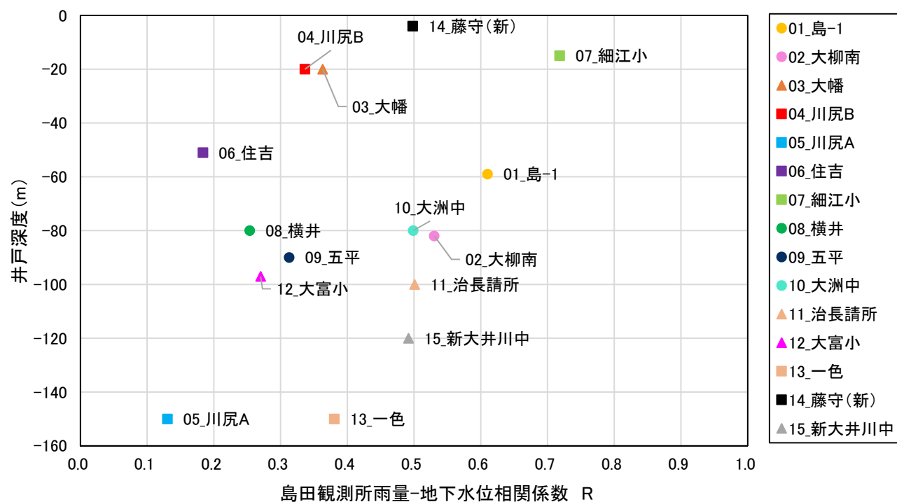
図 2.26 井戸深度と地下水位・島田観測所雨量の相関関係
