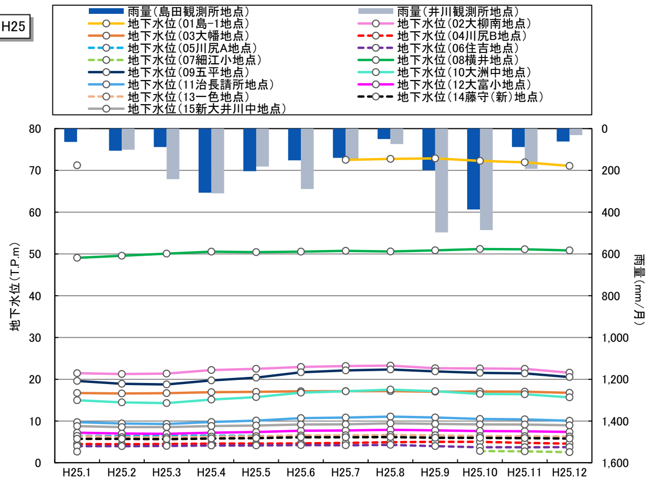
図 2.22 (2) 地下水位と降水量の経年変化 (H24, H25)
