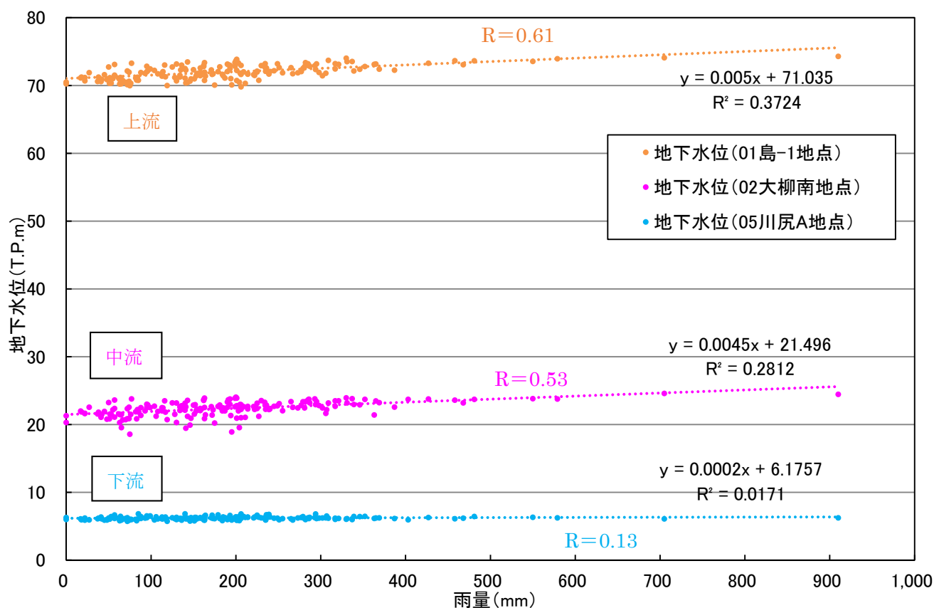
図 2.23 (1) 地下水位と島田観測所雨量の相関関係
