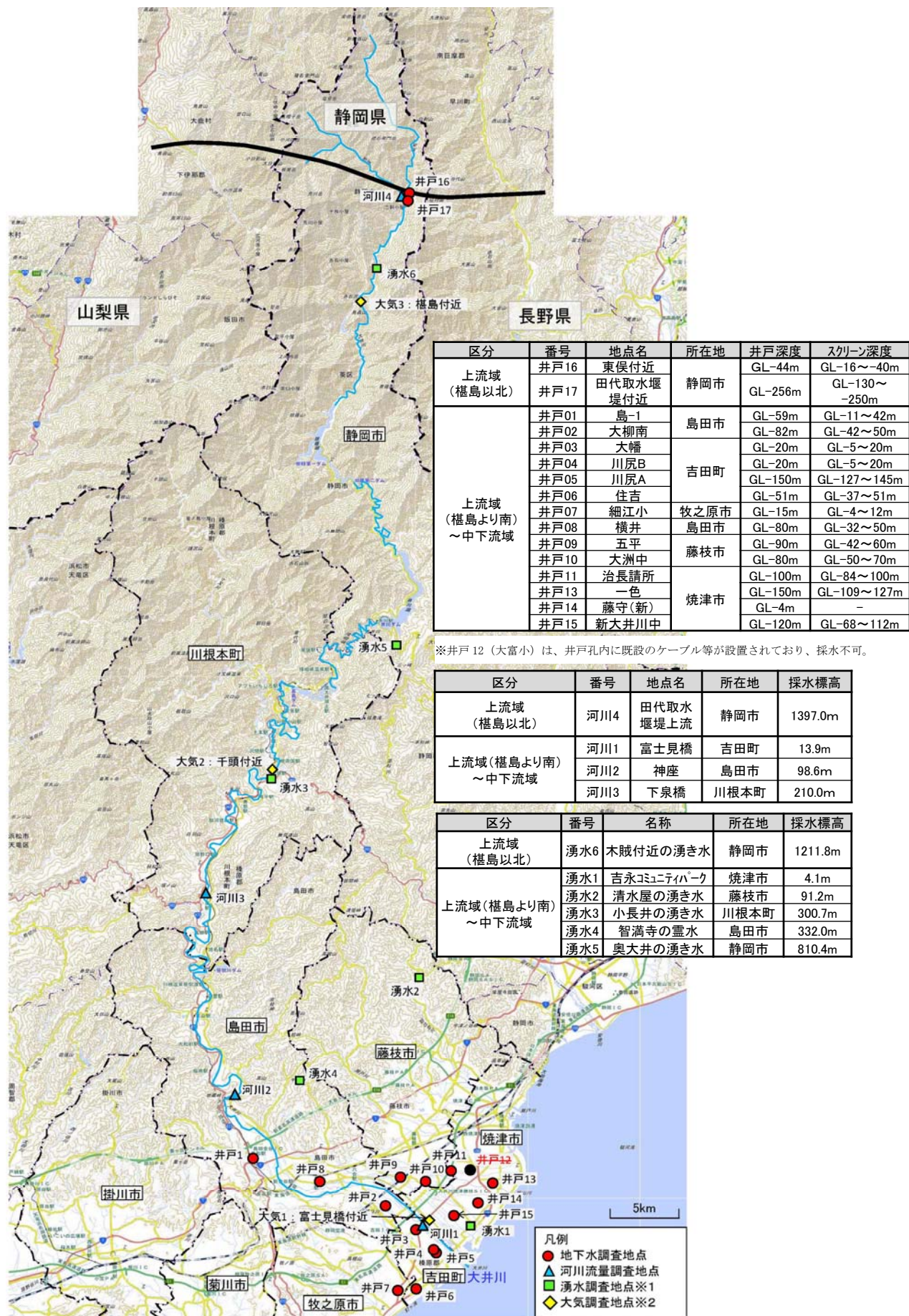
図 2.2.9 成分分析の測定地点
