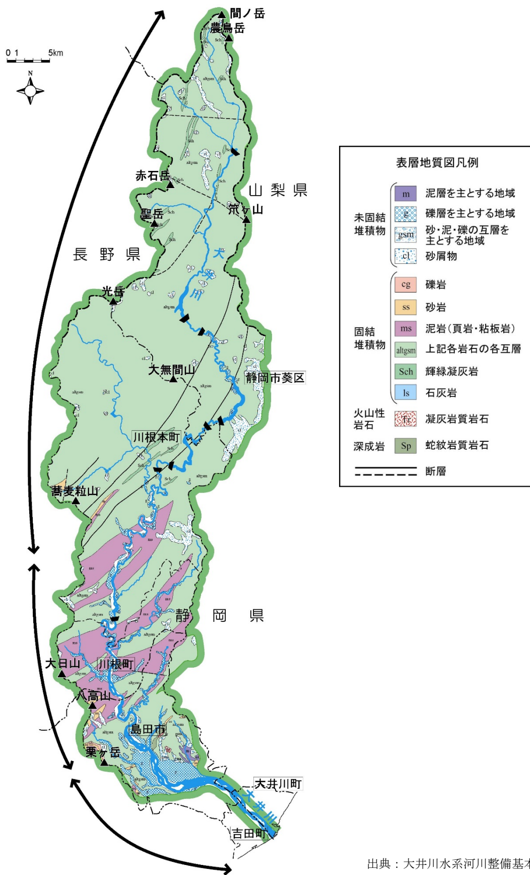
図 2.4 大井川流域の地質図
