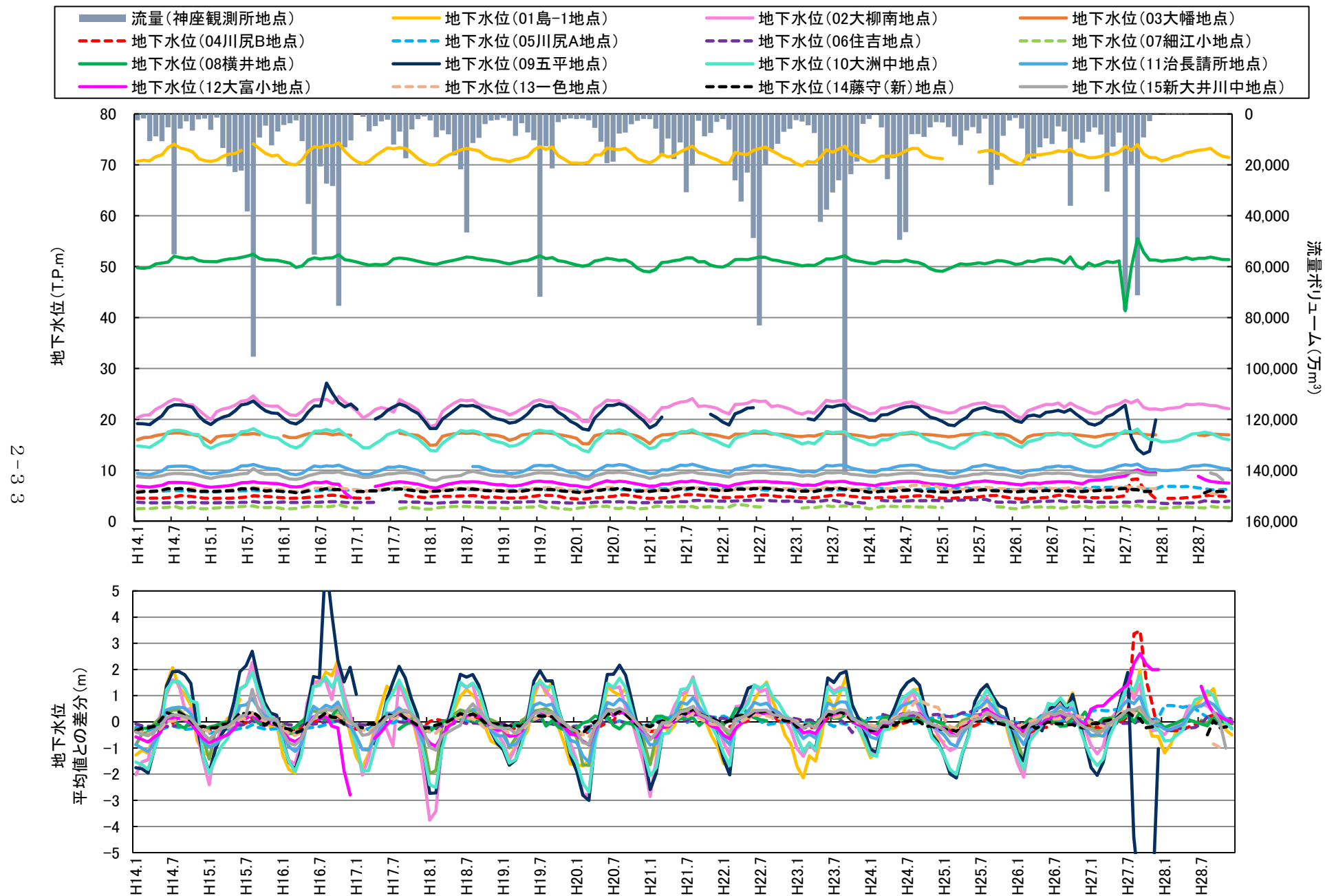
図 2.24 地下水位と神座地点流量の経年変化 (H14～H28)
