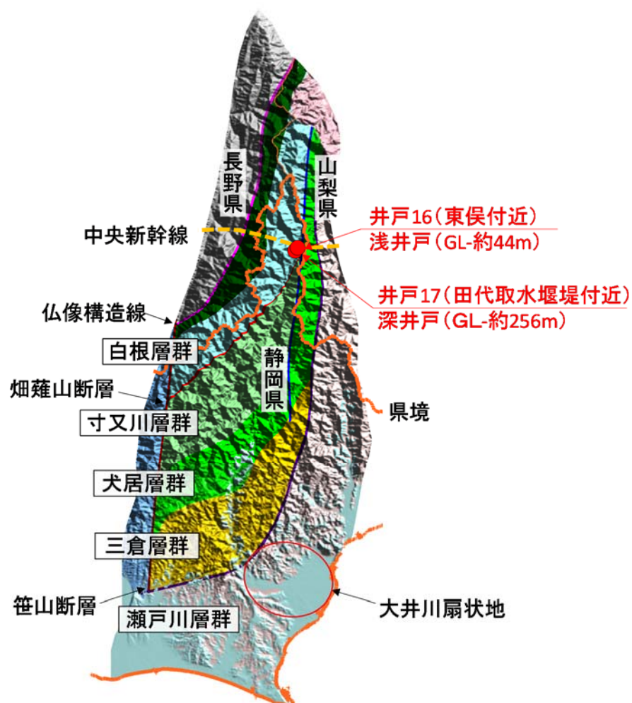
図 2.28 大井川流域の地層分布と上流域（樺島以北）の観測井の位置図
