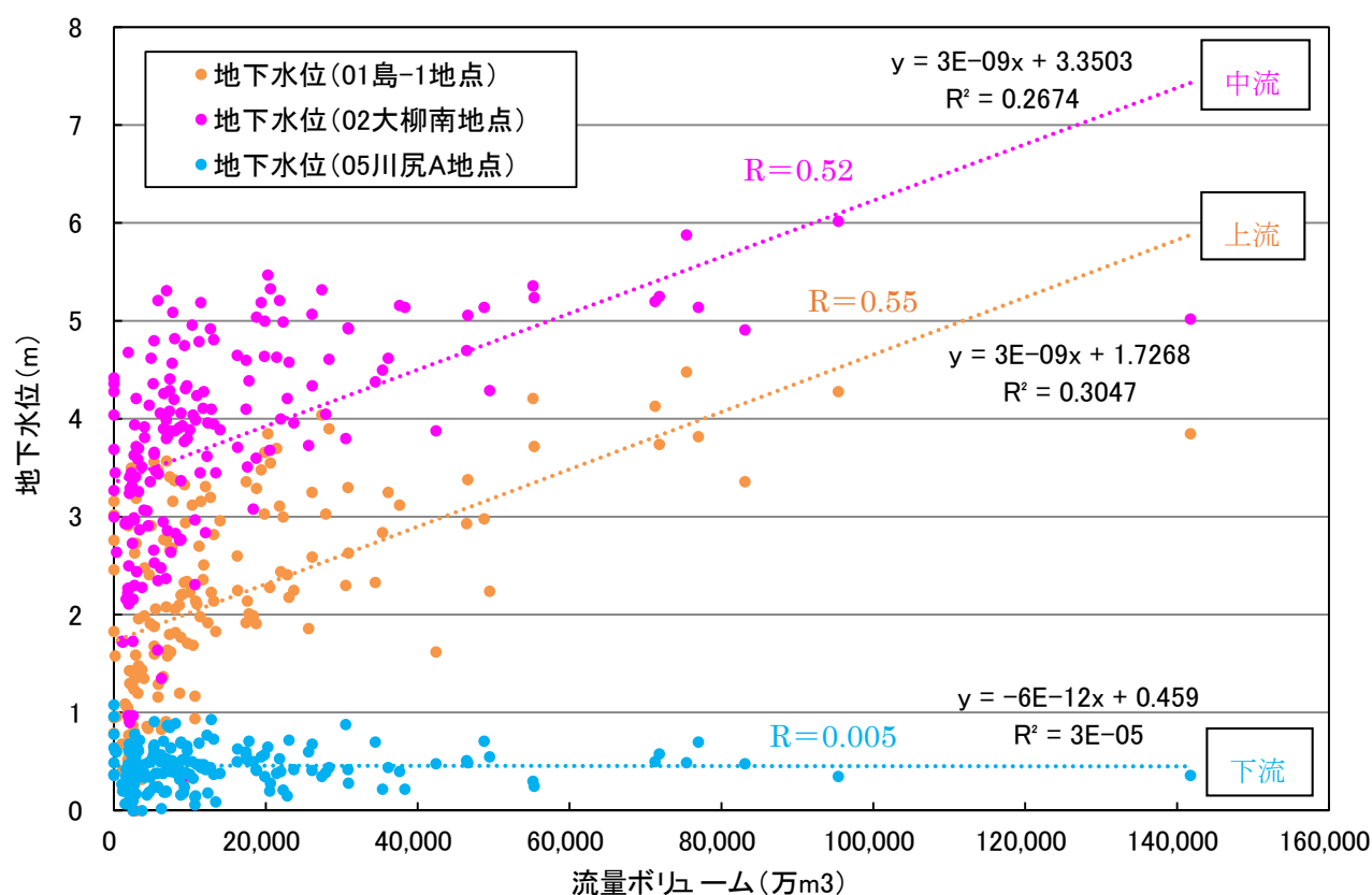
図 2.25 (1) 地下水位と神座地点流量の相関関係
