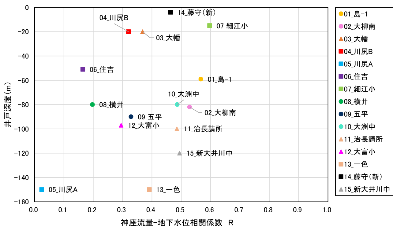
図 2.27 井戸深度と地下水位・神座地点流量の相関関係
