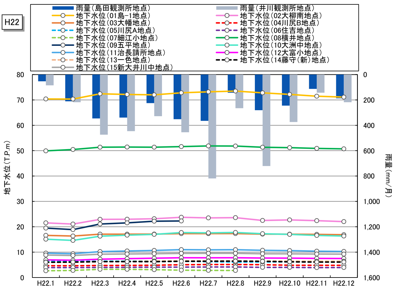
図 2.22 (1) 地下水位と降水量の経年変化 (H20、H21)
