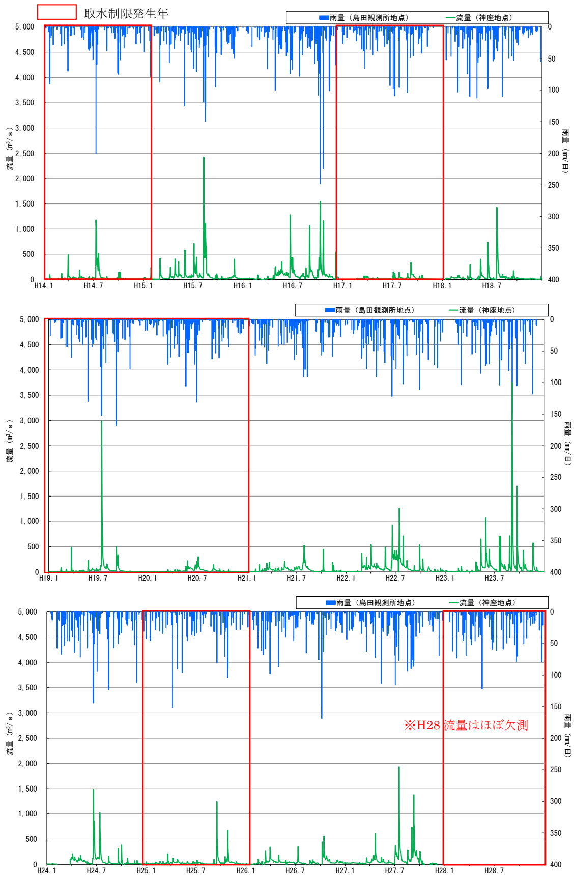
図 2.7 下流域における流量と降水量の経年変化
