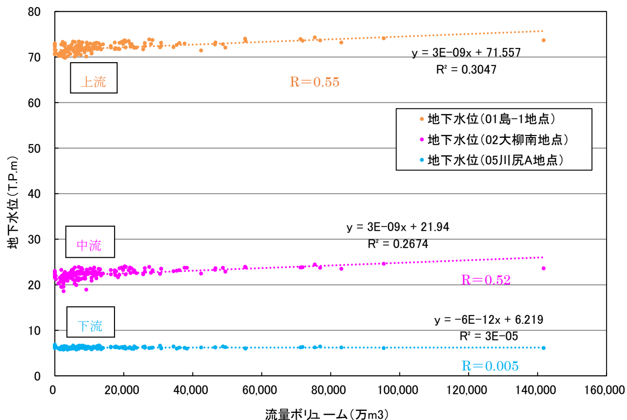
図 2.25 (1) 地下水位と神座地点流量の相関関係
